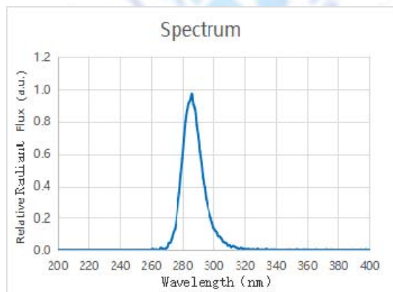
5) 光谱分布特性曲线
