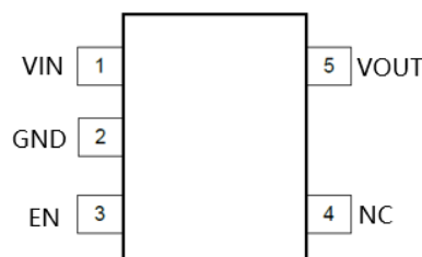
SOT23-5L/SOT-353
