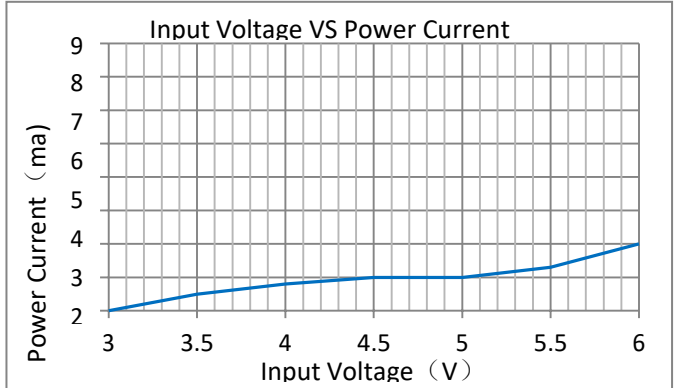
图4 : Input Voltage VS.Power Crrnt
