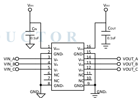
图 2. \pi 130x3x 应用简图
