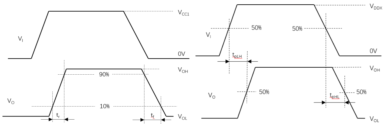
图 9. 传输时间波形测量
