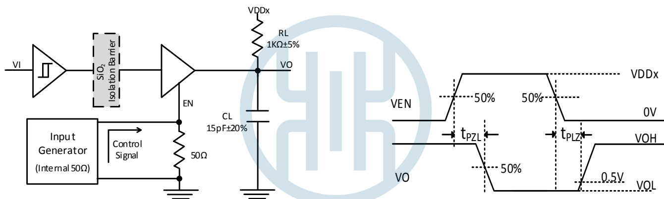
图 11. t_{PZL}/t_{PLZ} 测试线路
