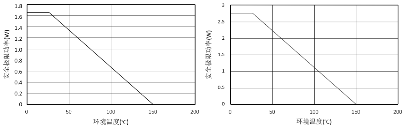
图 5.热降额曲线，依据 DIN V VDE V 0884-11 的安全限值与环境温度的关系(左: \pi 13xU3x ; 右: \pi 13xU6x )
