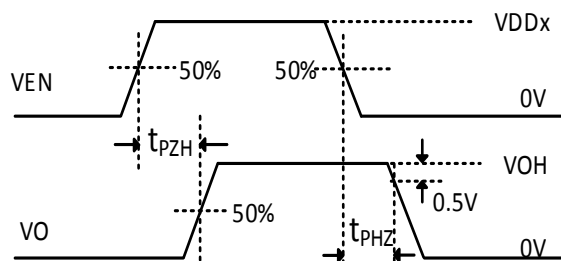
图 14. t_{PZH}/t_{PHZ} 测试波形
