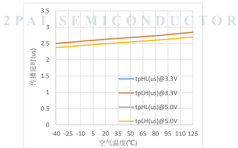
图 8. \pi 13xU6x 传输延时 vs. 空气温度
