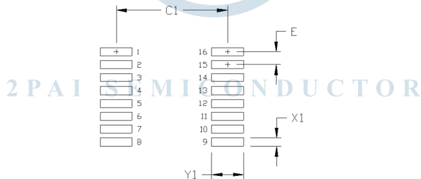
图 22. 16 引脚 SSOIC 封装 [16-Lead SSOP] 焊盘图案
