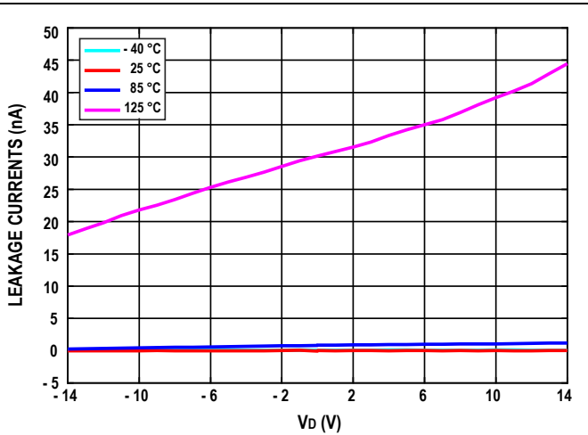
图5. 导通状态下，不同温度的漏端漏电流和漏端电压的关系
