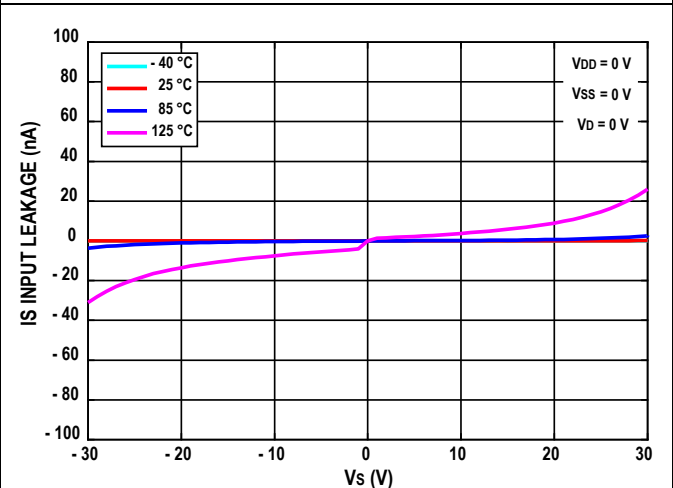
图4. 掉电状态下，不同温度的源电流和源电压关系
