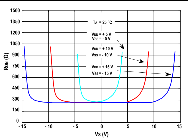
图1. 导通电阻和源(漏)电压的关系
