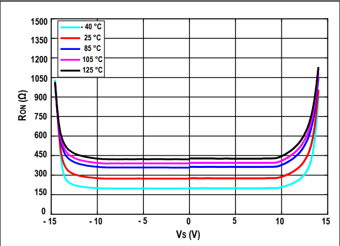
图2. 不同温度的导通电阻和源(漏)电压关系
