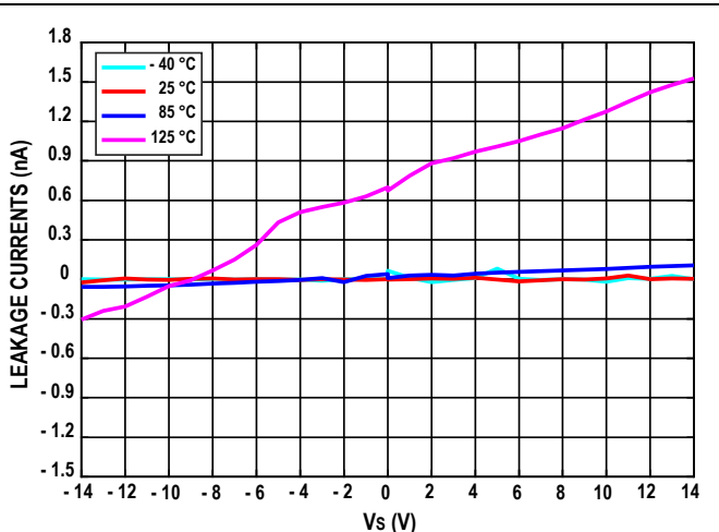
图3. 上电并关断状态下，不同温度的源电流和源电压关系
