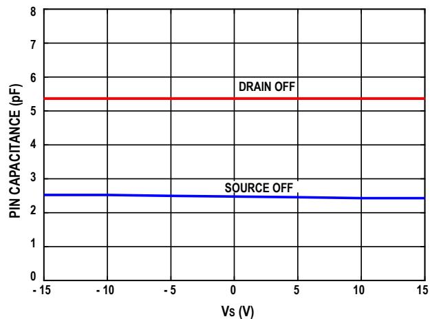
图10. 关断电容与源端电压关系
