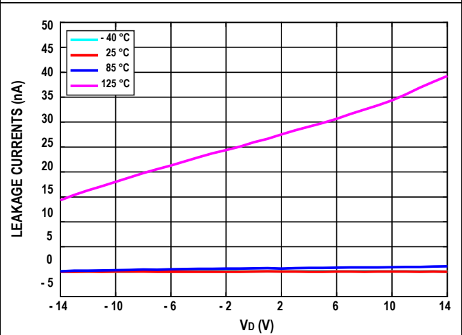
图6. 关断状态下，不同温度的漏端漏电流和漏端电压的关系
