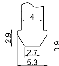
锁舌参考规格
