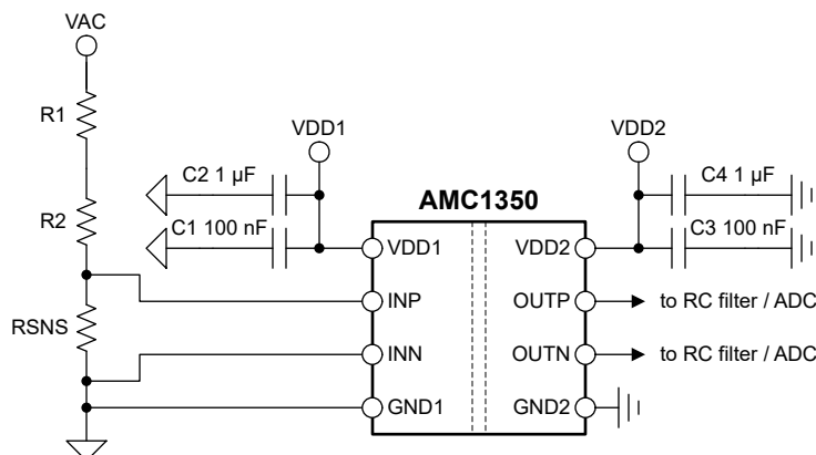
图 9-1. Decoupling of the AMC1350
