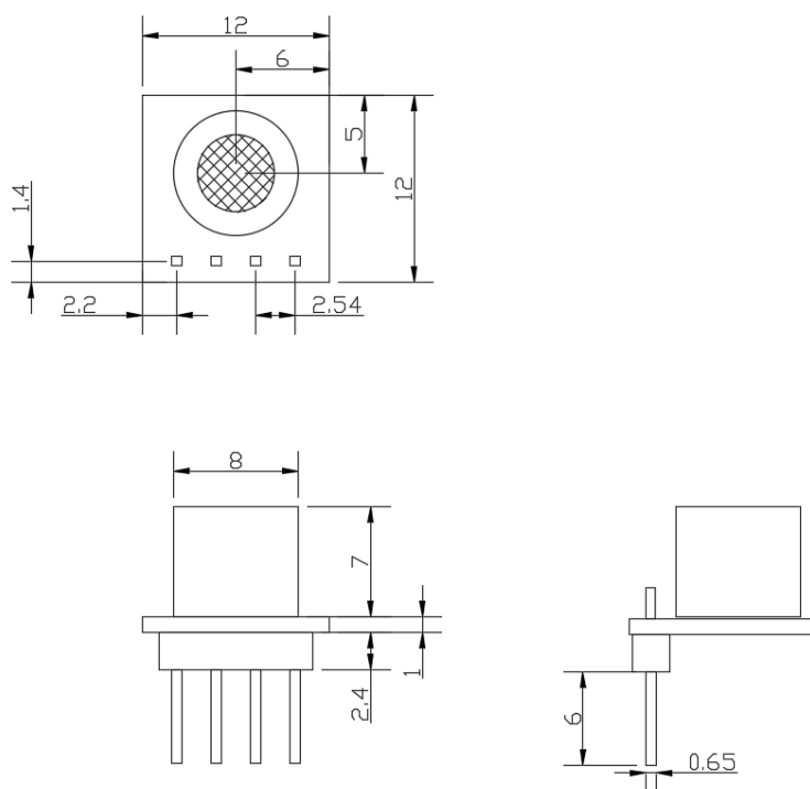
图 4. 产品尺寸图（单位：mm）
