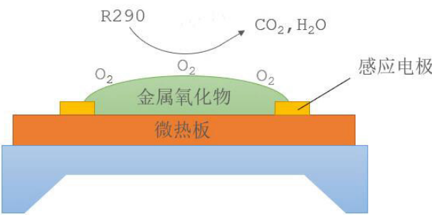
图 2. 原理示意图
