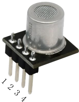
图 3. 引脚示意图
