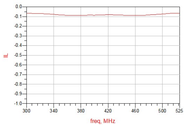
Figure 10. MHC0450L03 IL
