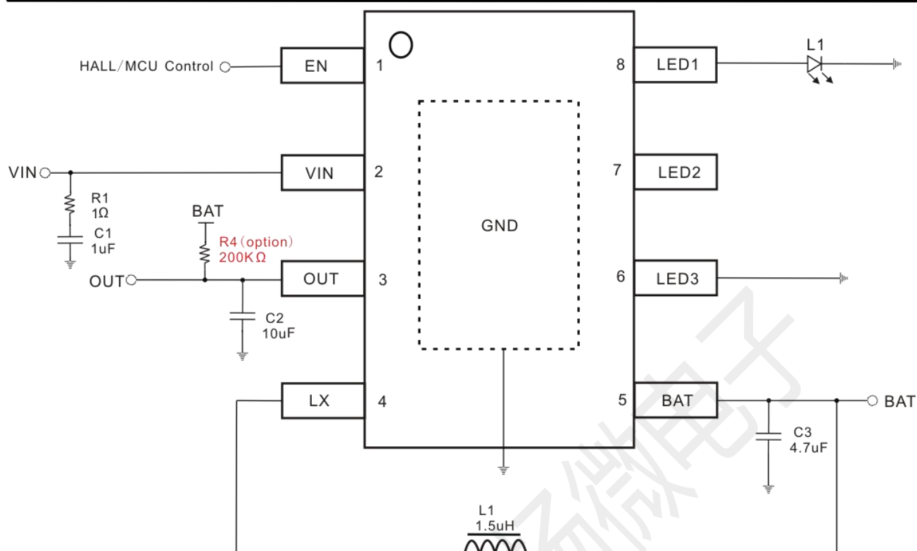
1 灯模式—2 (LED3 须接地)
