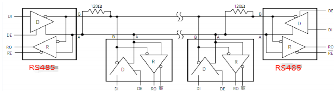
图 11 典型的 RS485 半双工通讯网络
