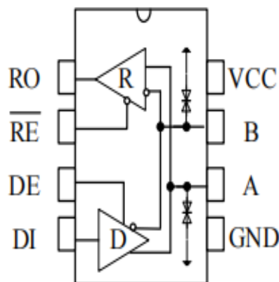
图 1 引脚分布图
