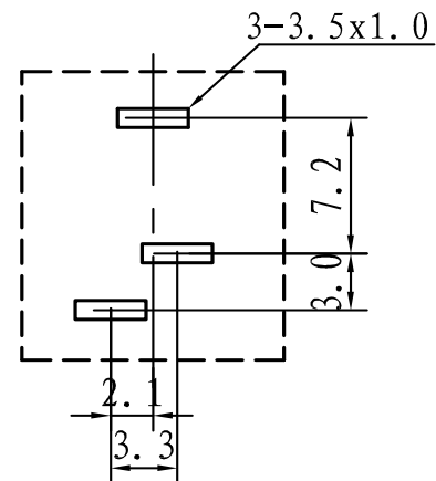
线路板安装尺寸示意图
