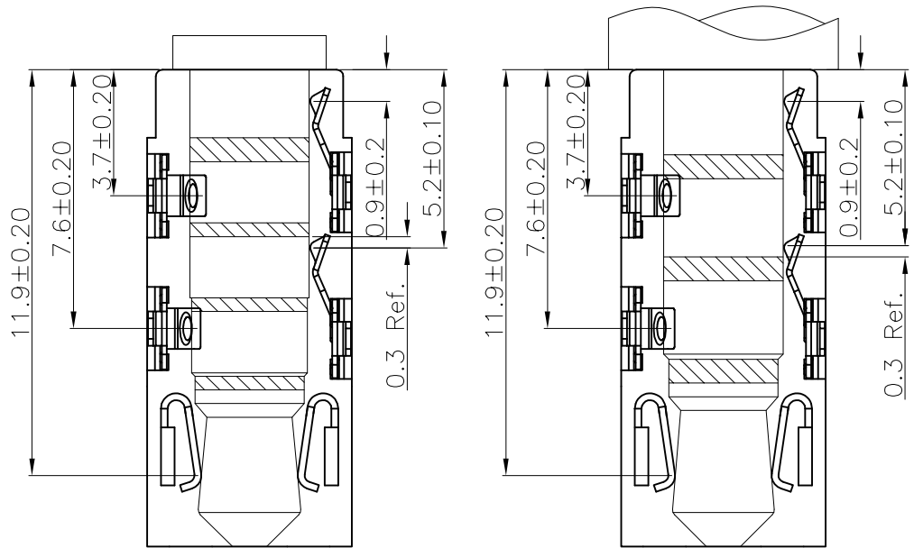
模拟5极插头接触状态 模拟4极插头接触状态
