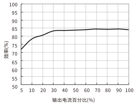
效率Vs输出负载(Vin=24V) URB2405YMD-10WR3
