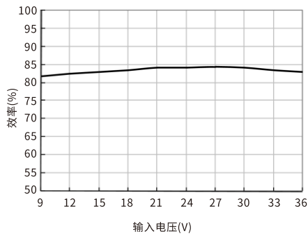
效率Vs输入电压(满载) URB2405YMD-10WR3
