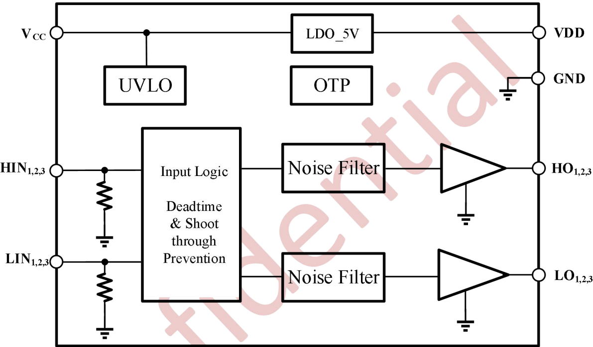
图 9-1 NSG0360 功能框图
