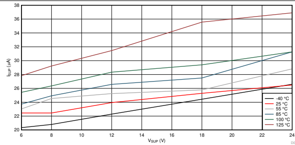
图 1. I_{SUP} vs V_{SUP} Sleep Mode
