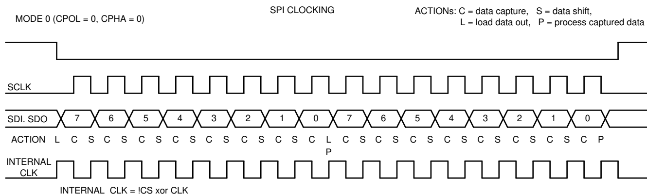
图 33. SPI Clocking
