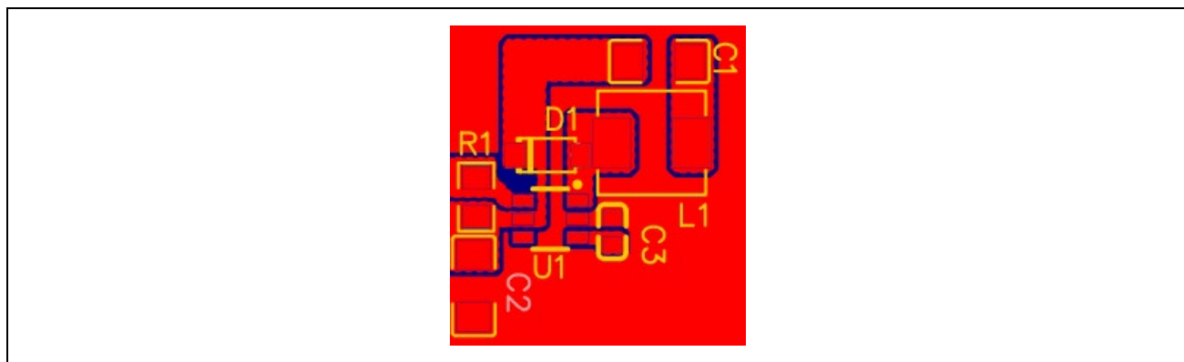
图 8.BUCK 型 SOT23-6 封装典型应用 PCB 参考布局
