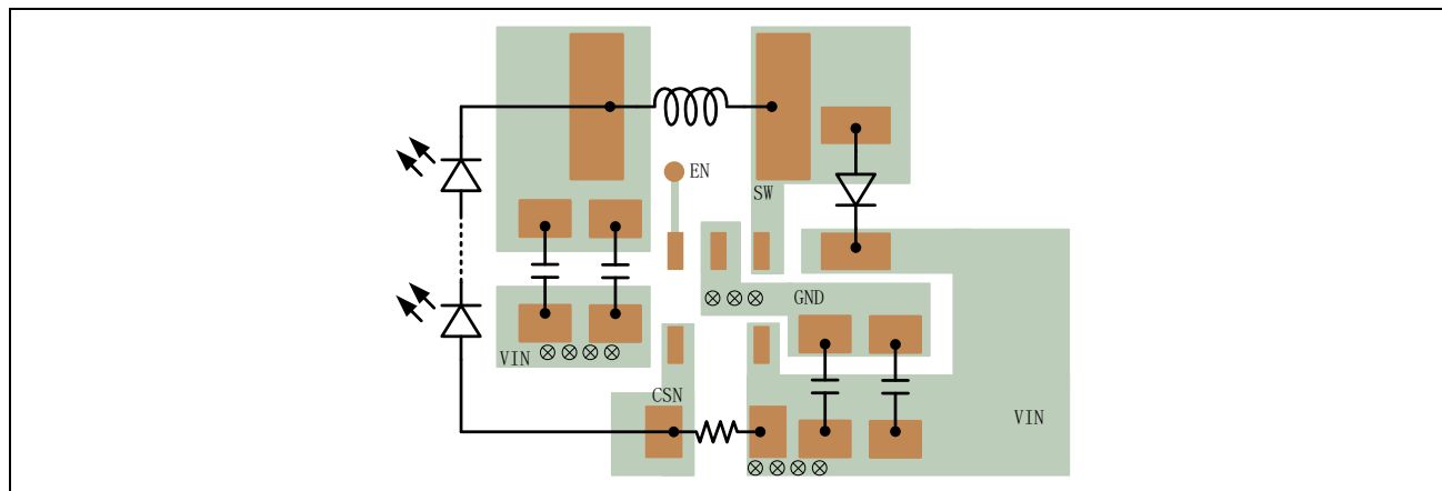
图 15.2 BUCK 型 SOT23-5 封装典型应用 PCB 参考布局
