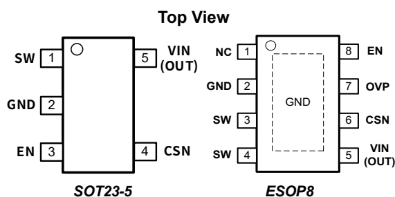
封装与引脚排列
