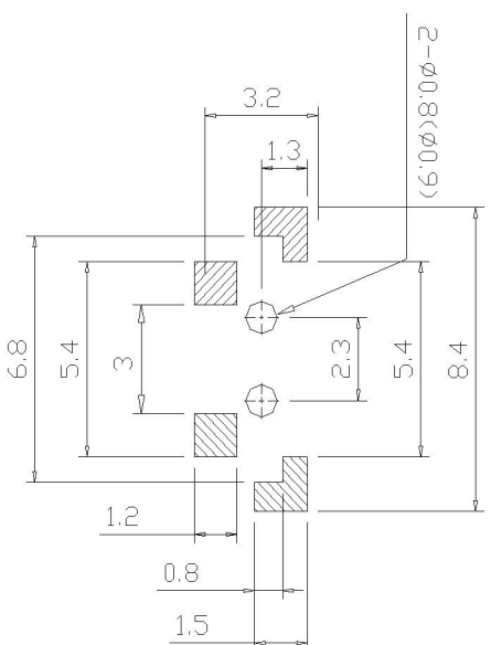
PCB. 焊接图
