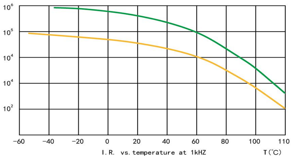
I. R. ( \text{M}\Omega ) 绝缘电阻变化
