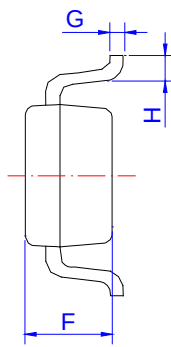
SOT-23-3L
