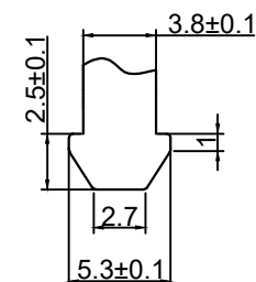
锁舌参考规格
