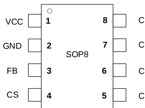
图 2 管脚封装图
