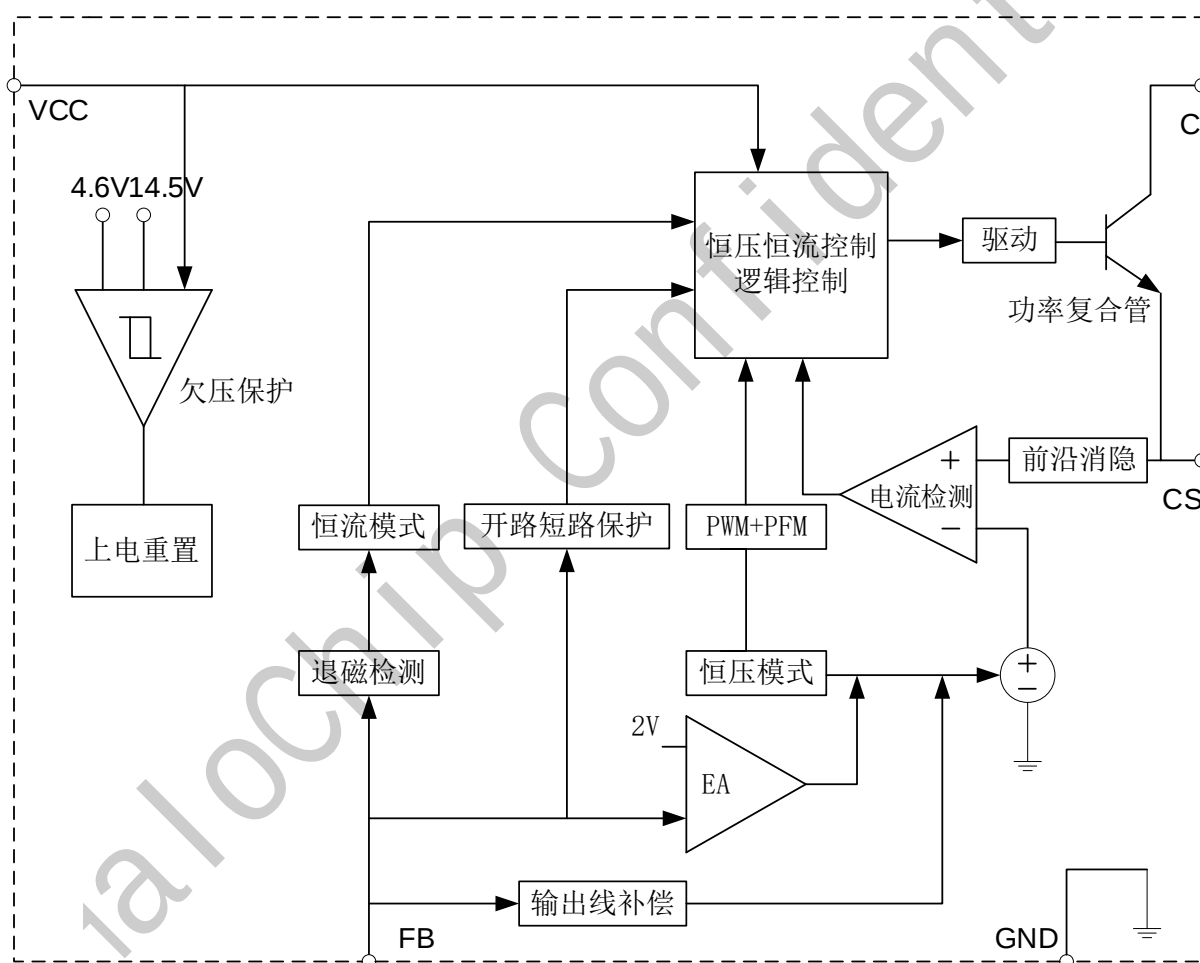
图 3 GP8691X 内部框图
