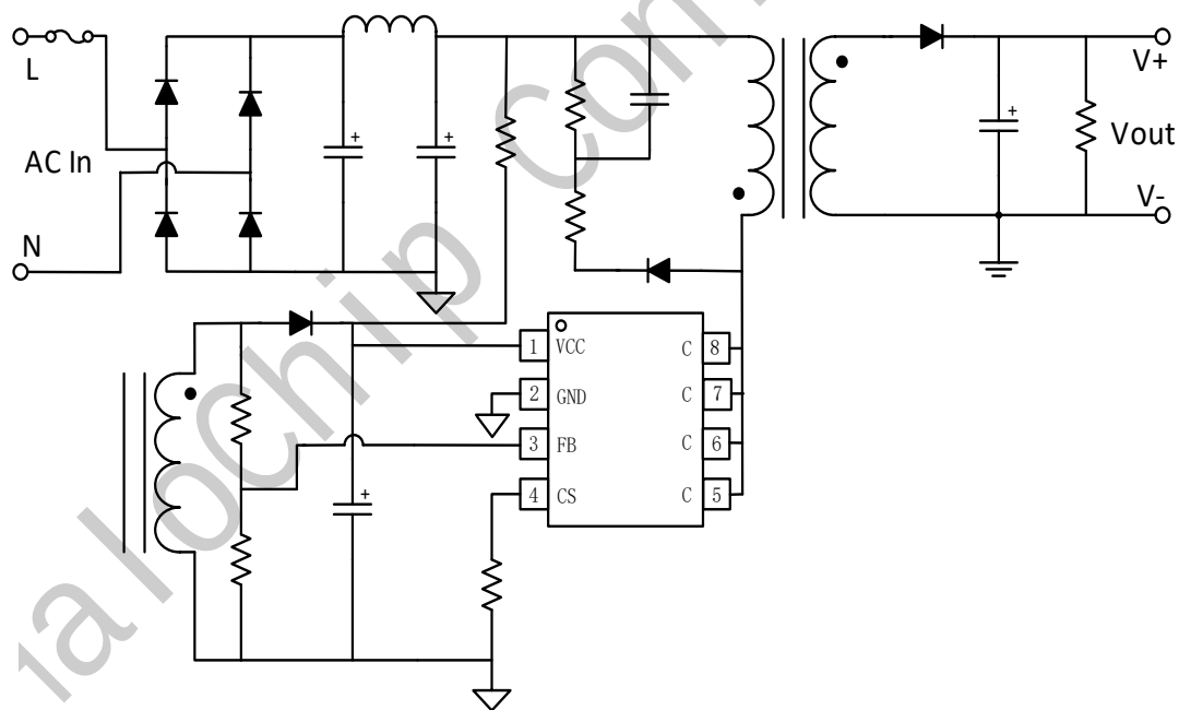
图 1 GP8691X 典型应用图
