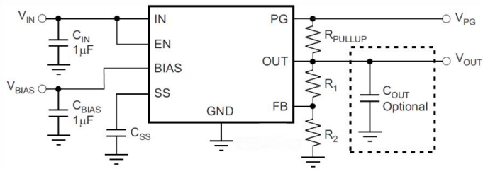
图 1 LKP21190QF 系列典型应用电路图
