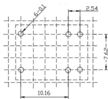
◆ 印刷线路板加工尺寸 PCB Outline Dimension Bottom View
