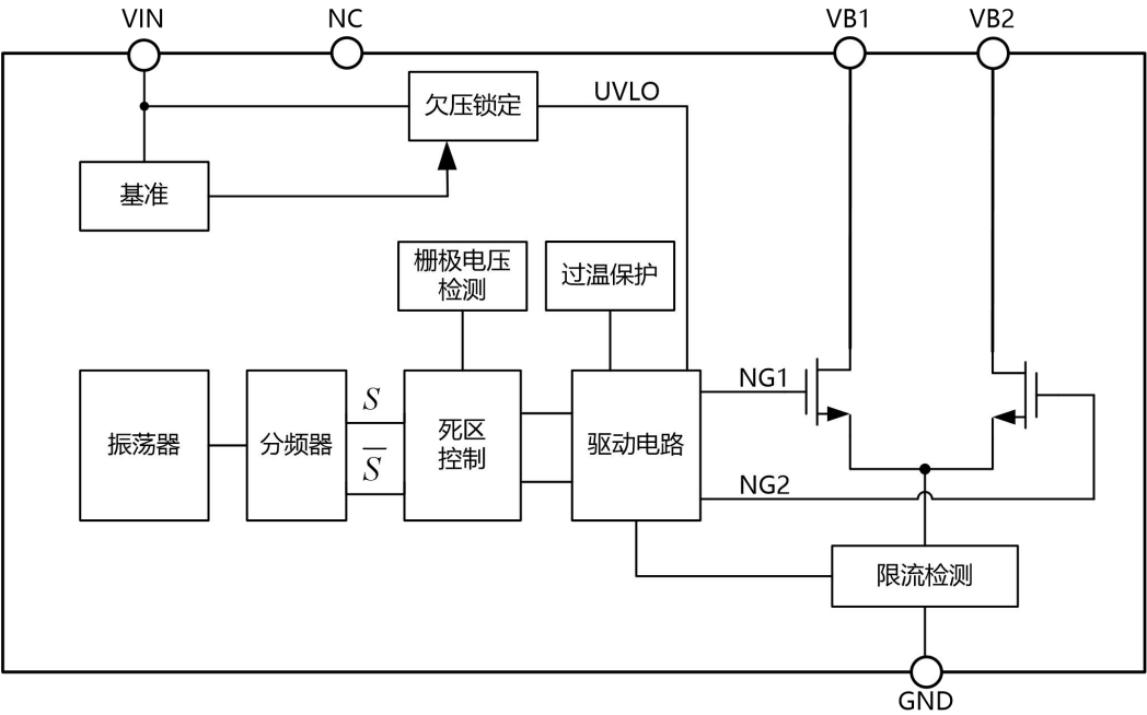
图 8.1 原理示意图
