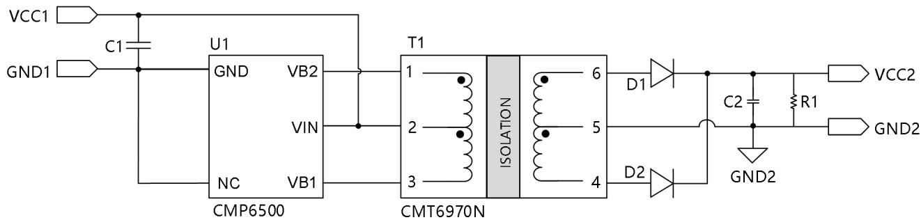
图 8.2 设计原理图
