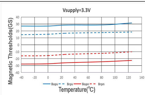
X 轴磁场阈值 VS 工作温度 @VDD=3.3V
