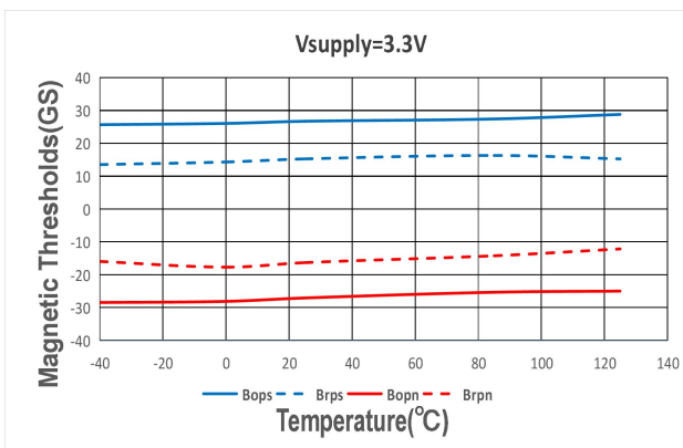
Y 轴磁场阈值 VS 工作温度 @VDD=3.3V
