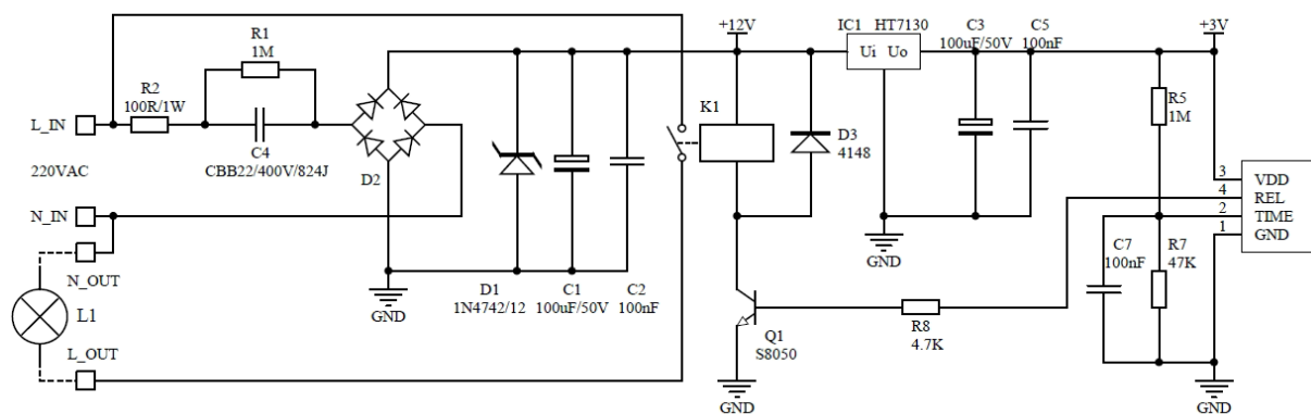
SY-DP-36BP4数字热释电典型应用电路
