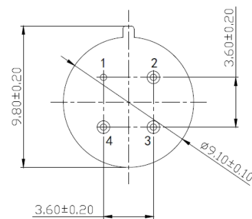
底视图
