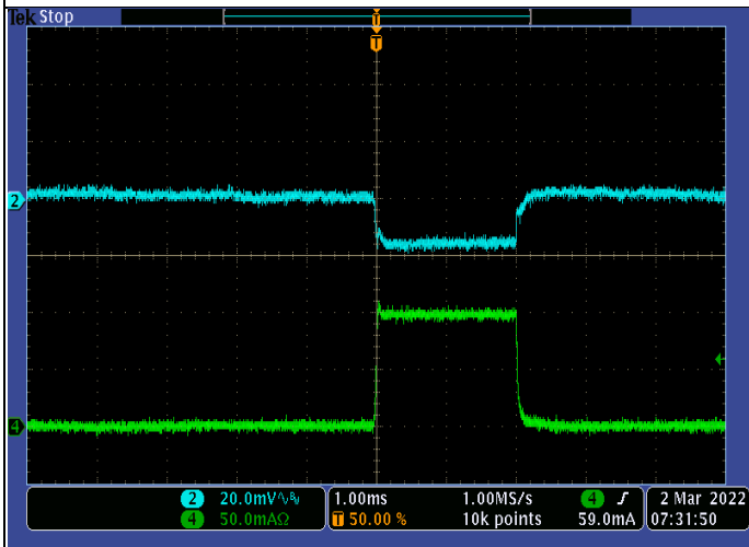
Fig 9. 负载瞬变
