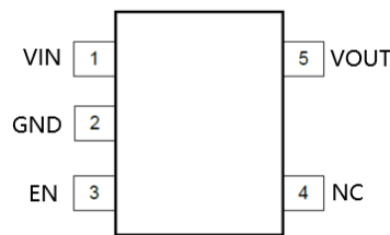
SOT23-5L
