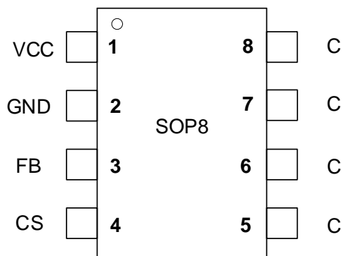
图 2 管脚封装图
