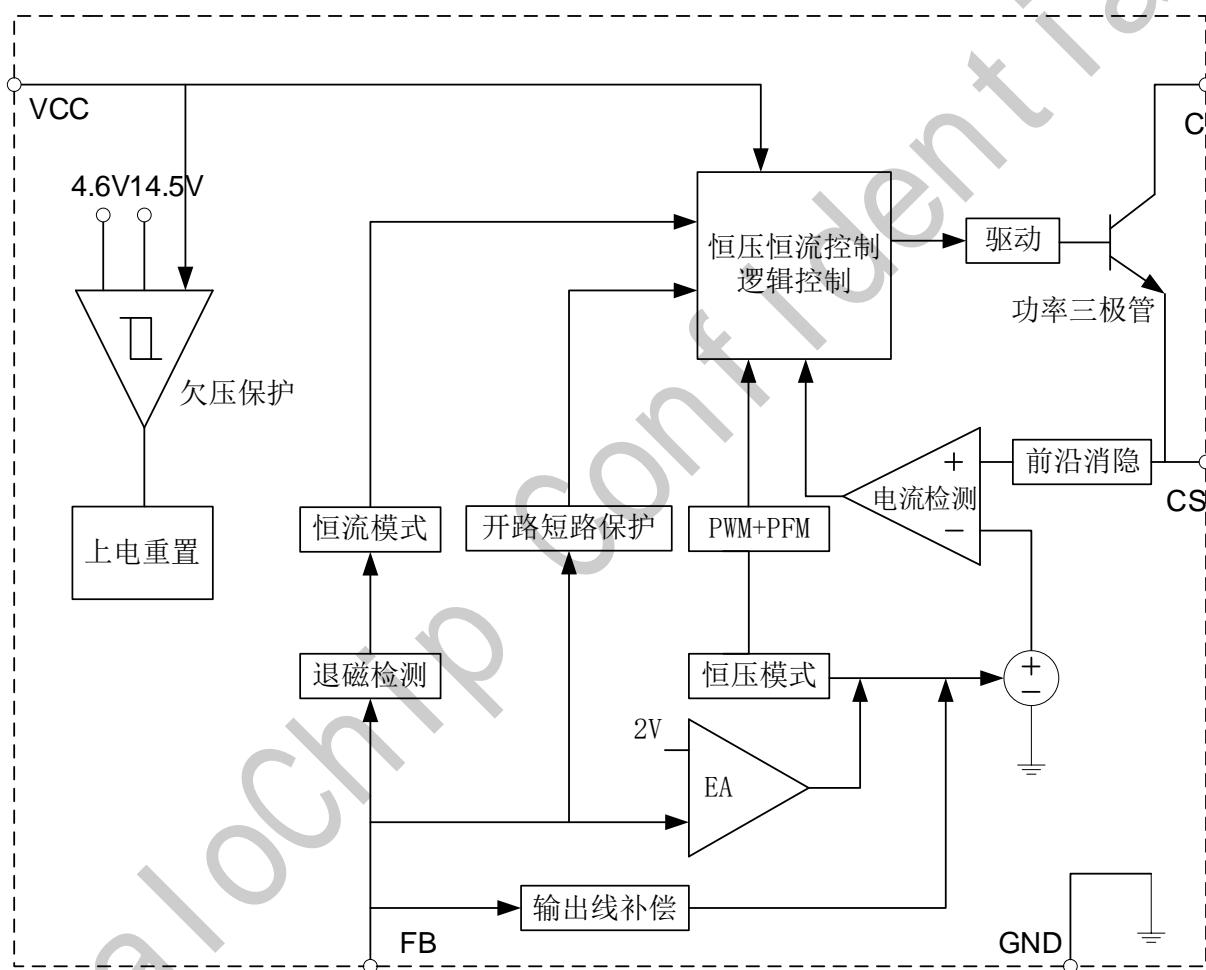
图 3 GP8615X 内部框图
