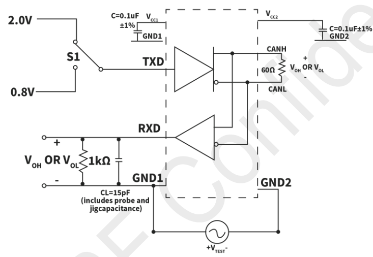
图 14. 共模瞬态抑制(CMTI)测量电路
