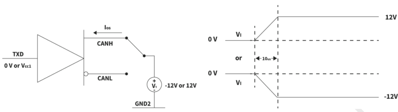
图 13. 驱动器短路电流测试电路及波形
