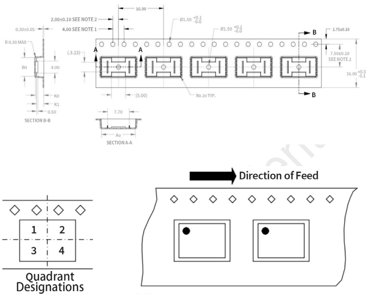
图 22. CMT10XXX SOIC8 卷带信息
