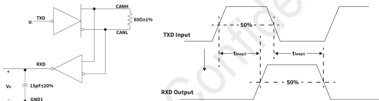
图 11. t_{\text{Loop}} 测试电路和电压波形
