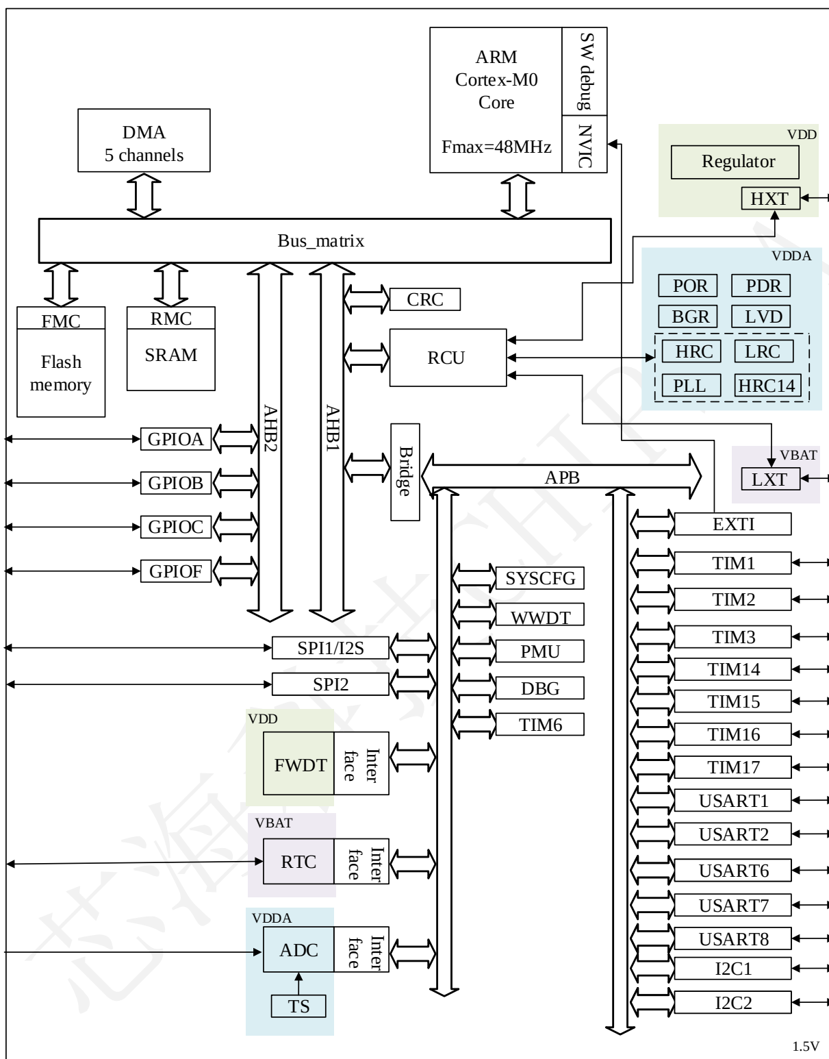
图 1 模块框图
