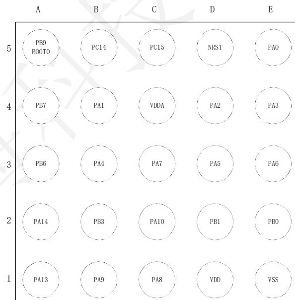
图 5 WLCSP25 封装引脚图（marking side）
