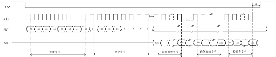
图 5-2 SPI 读时序
