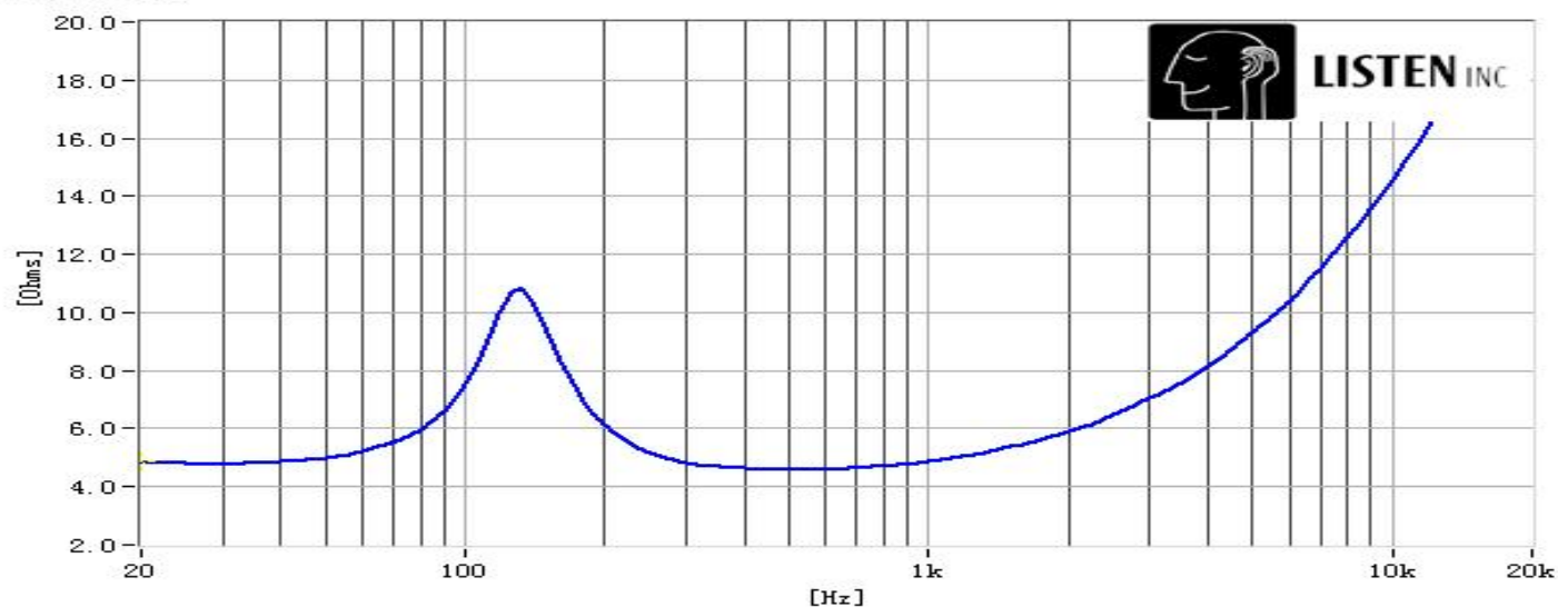
阻抗曲线
