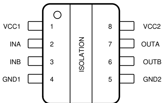
图 4-1. ISO6520 D Package 8-Pin SOIC Top View
