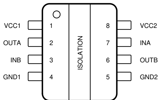
图 4-2. ISO6521 D Package 8-Pin SOIC Top View
