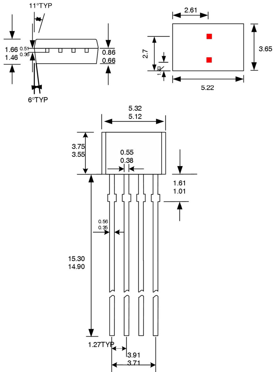
4-脚 VB 封装
