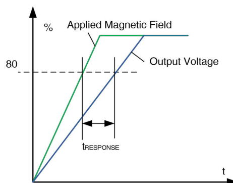
图2 响应时间
