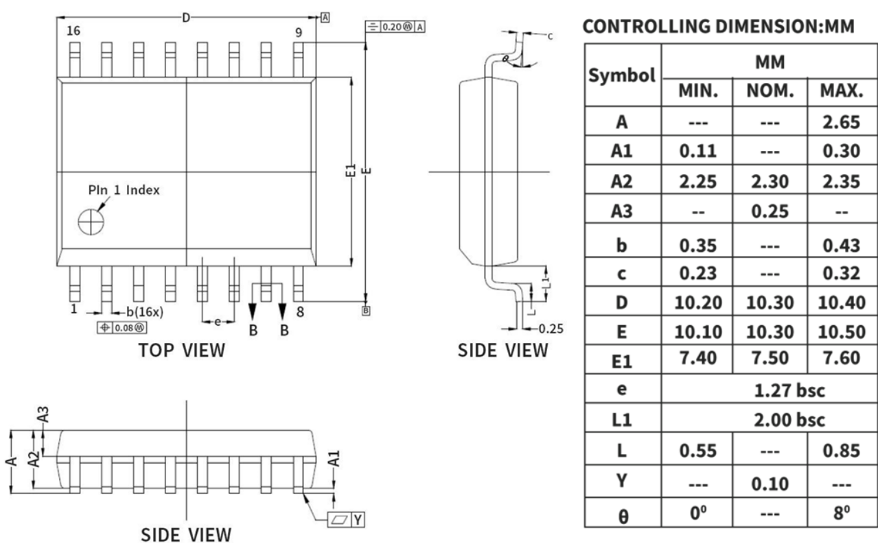
图 18. CMT10XXX SOIC 16 封装外形和尺寸
