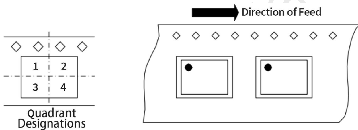
图 22. CMT10XXX SOIC8 卷带信息
