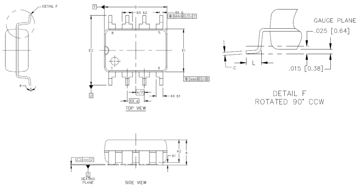
图 20. CMT10XXX DUB8 封装
