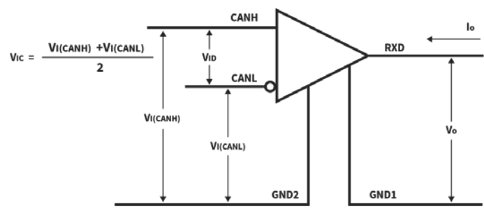
图 8. 驱动测试电路以及电压波形
