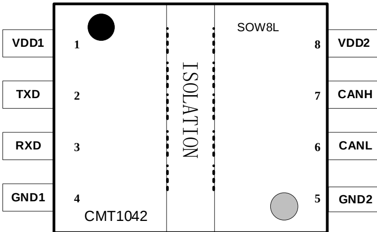
图 2. CMT1042W / CMT1052W 引脚图
