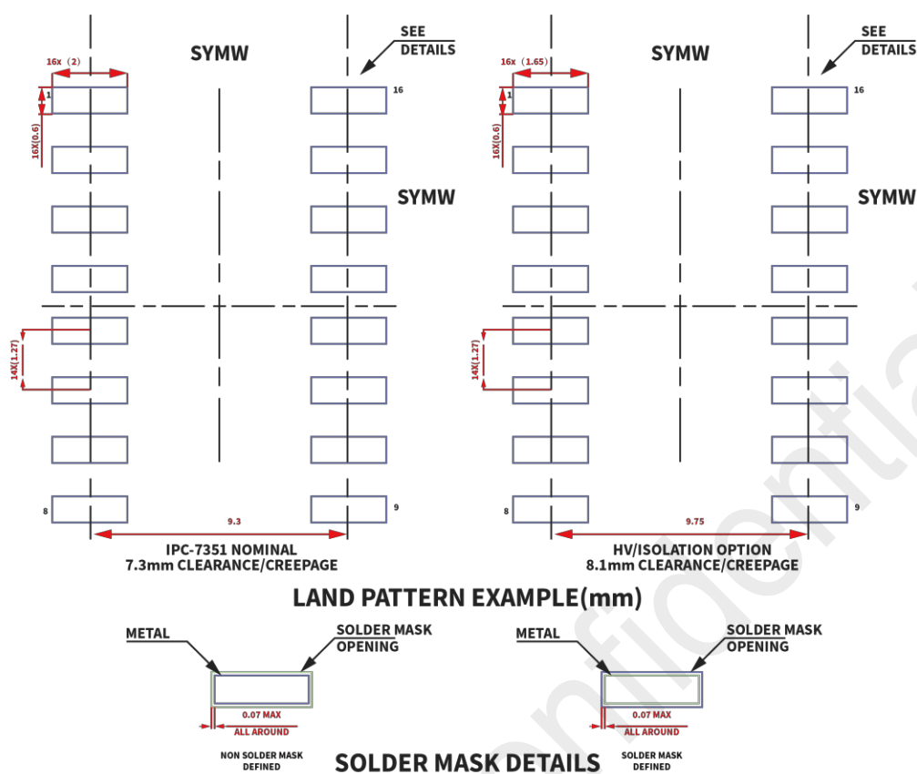
图 19. CMT10XXX SOIC-16 封装板布局示例
