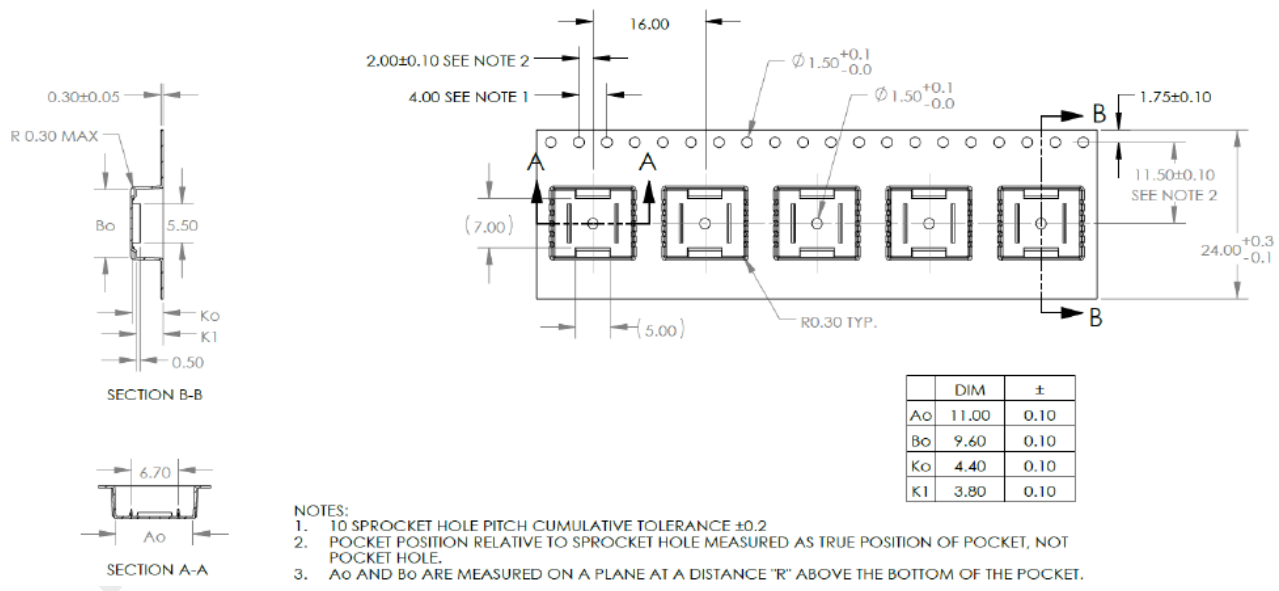
图 24. CMT10XXX DUB8 卷带信息
