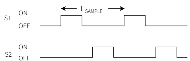
图 29 S1 和 S2 开关时序
