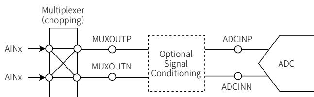
图 31 外部斩波
