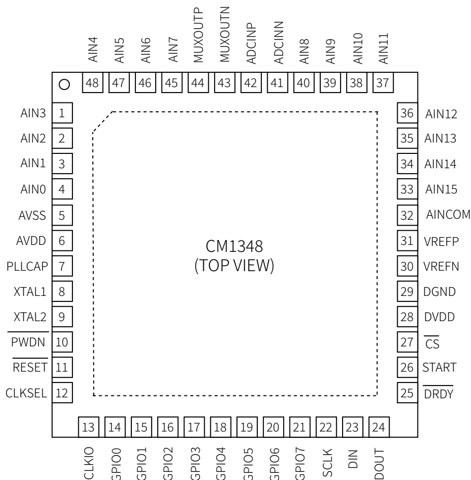
图 1 管脚示意图
