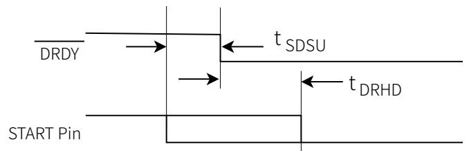
图 44 START 管脚和 \overline{\text{DRDY}} 时序
