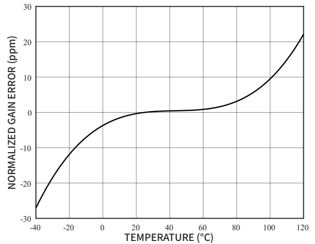
图 15 增益错误 vs 温度
