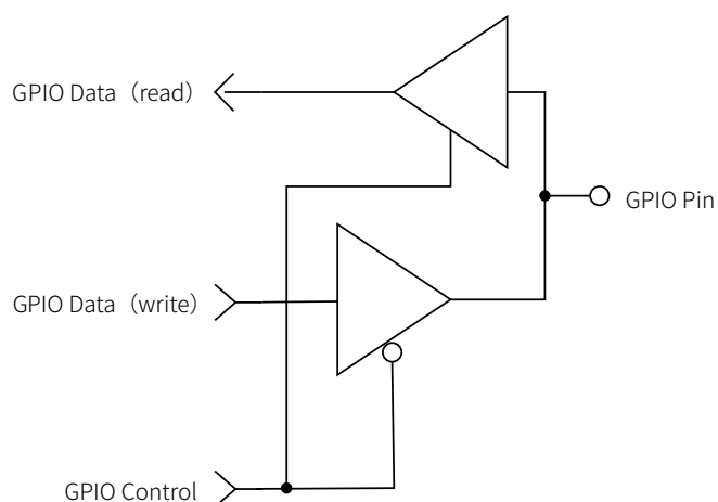
图 39 GPIO 端口管脚
