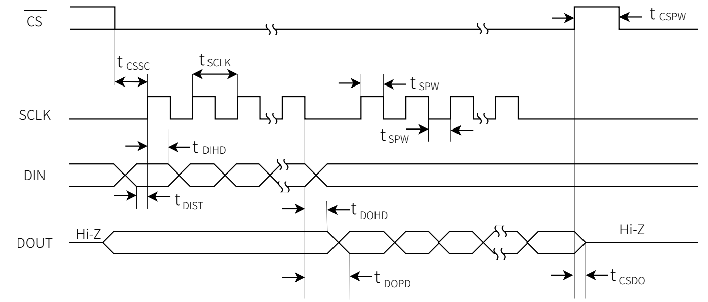
图 2 串行接口时序
