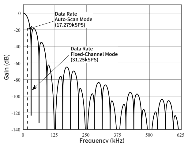
图 34 频率响应, DRATE[1:0]=10
