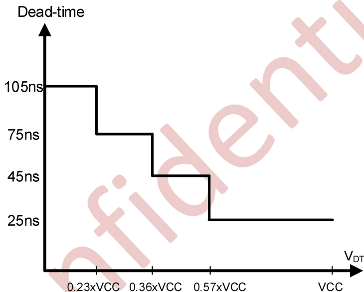
图 10-6 NSA2092 中死区时间与 V_{DT} 的关系
