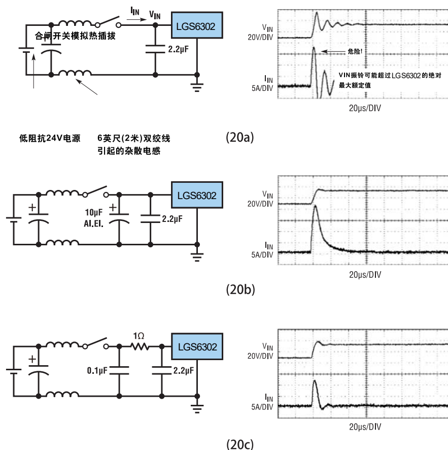
Figure 19. 精心选择的输入网络可防止输入电压过冲并确保 LGS6302 连接到带电电源时可可靠运行
