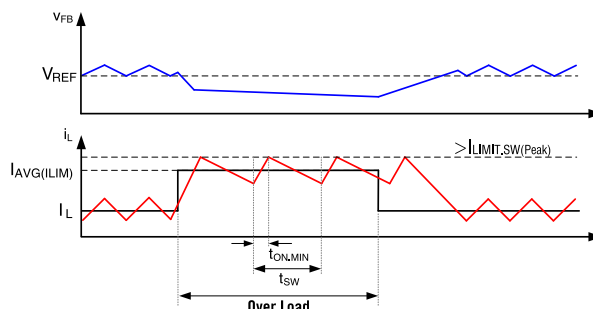
图 7. BOOST 输出过流于 M_{top} 行为描述
