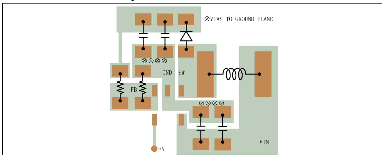
Figure 20.2 电路推荐 SOT23-5 封装 PCB 布局举例
