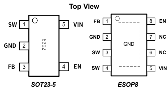
封装与引脚排列
