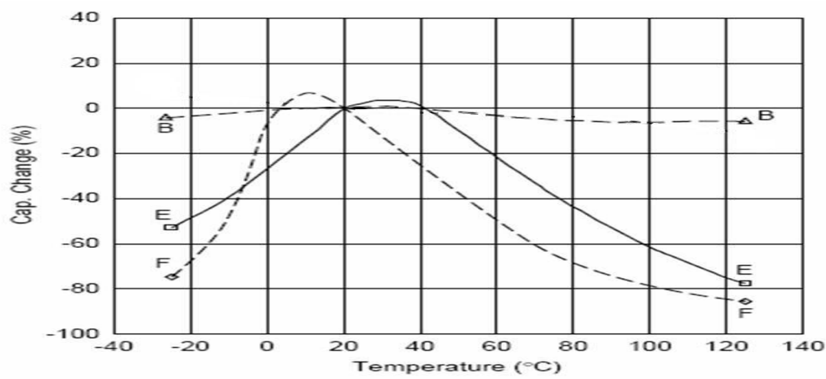
电容量特性曲线图
