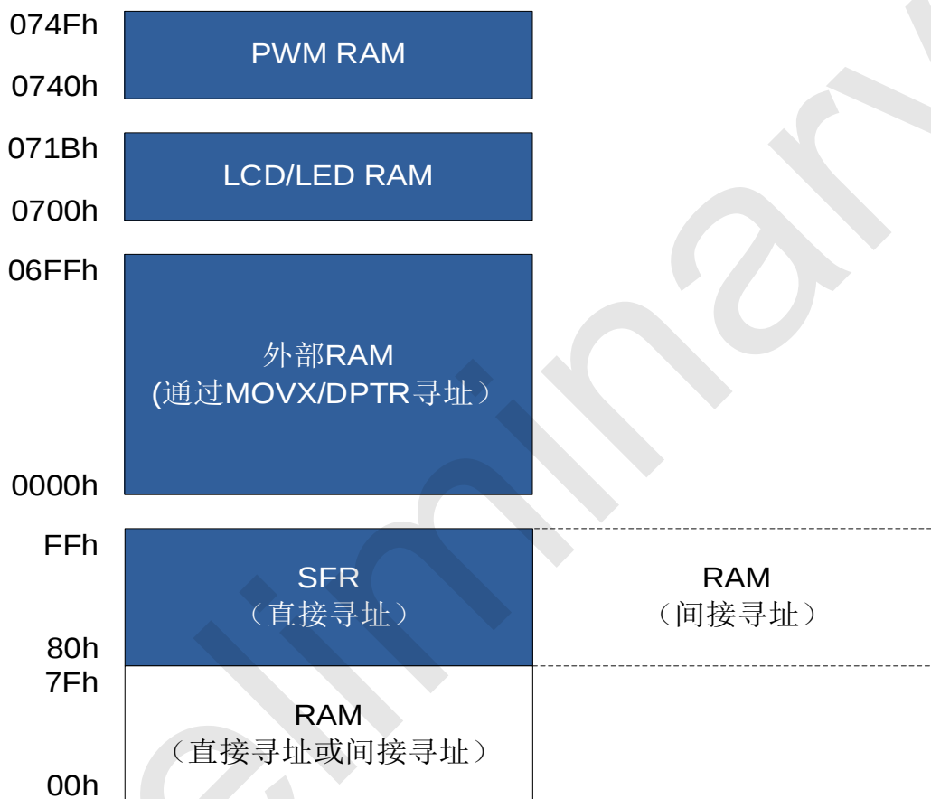
SRAM 结构图
