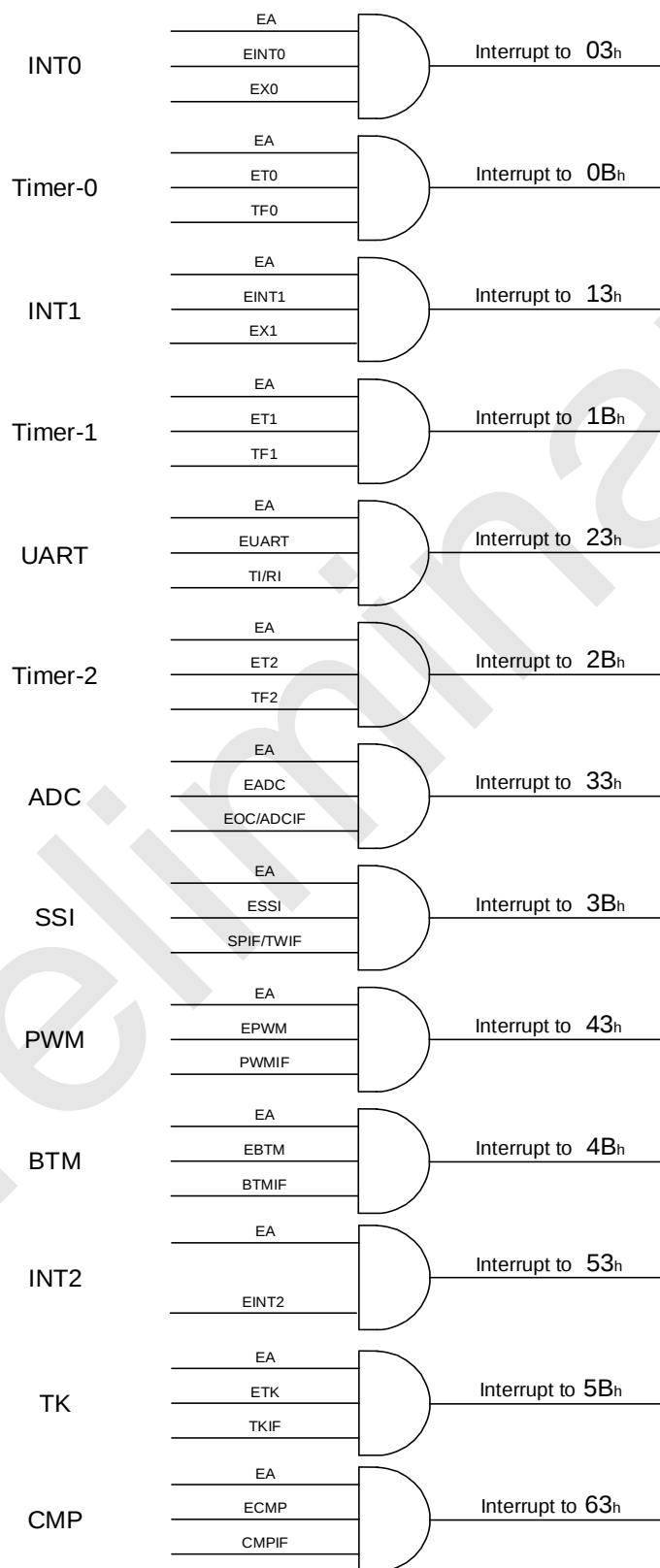
SC92F859X 中断结构和向量
