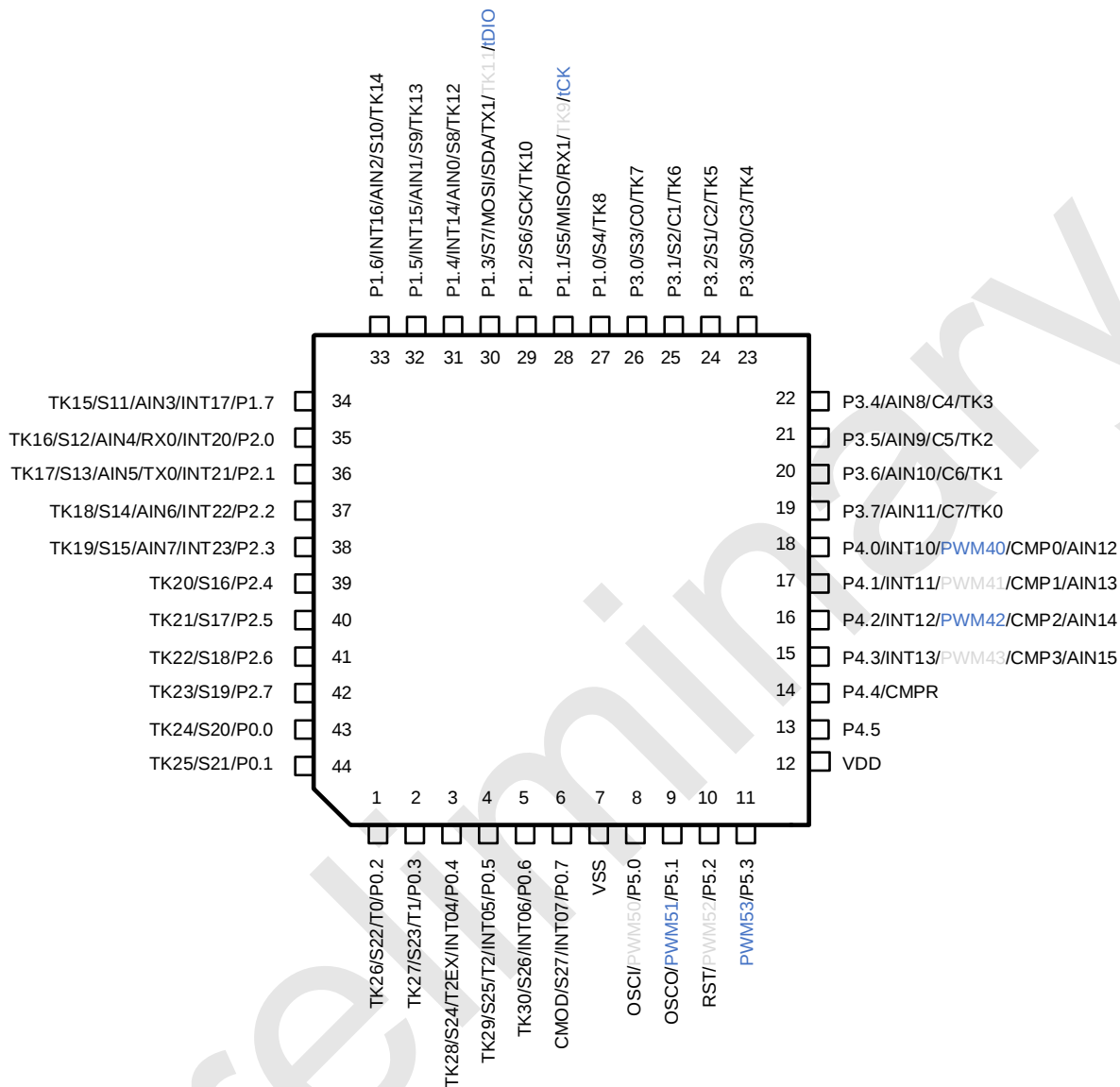
44PIN 管脚配置图
