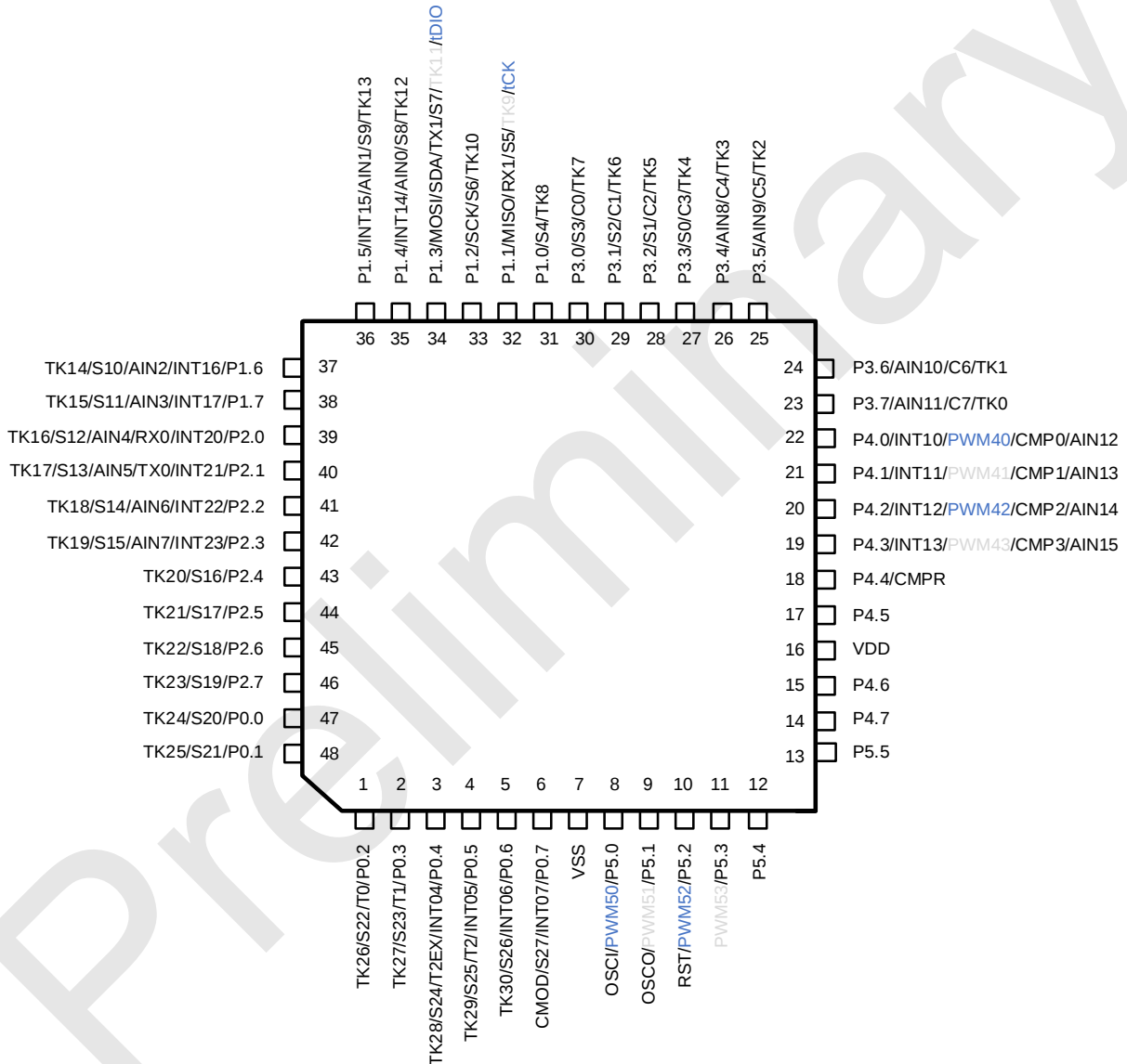
48PIN 管脚配置图
