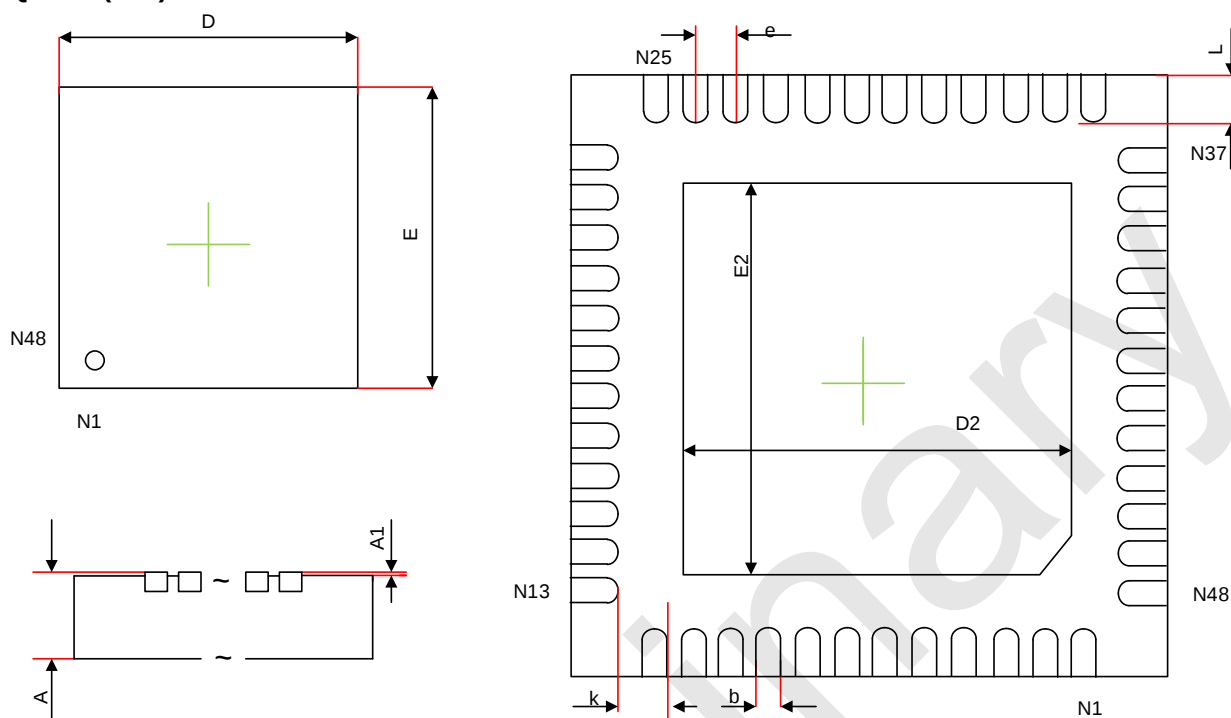
QFN48 (7X7)外形尺寸
