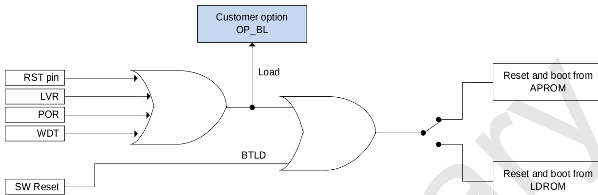
SC92F859X 复位后启动区域切换示意图
