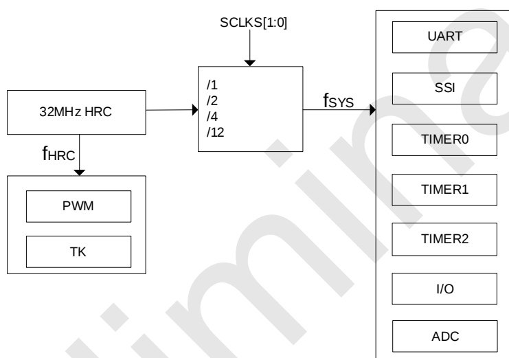
SC92F859X 内部时钟关系
