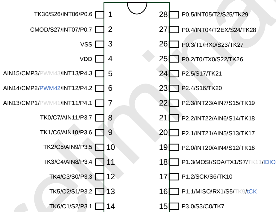
28PIN 管脚配置图
