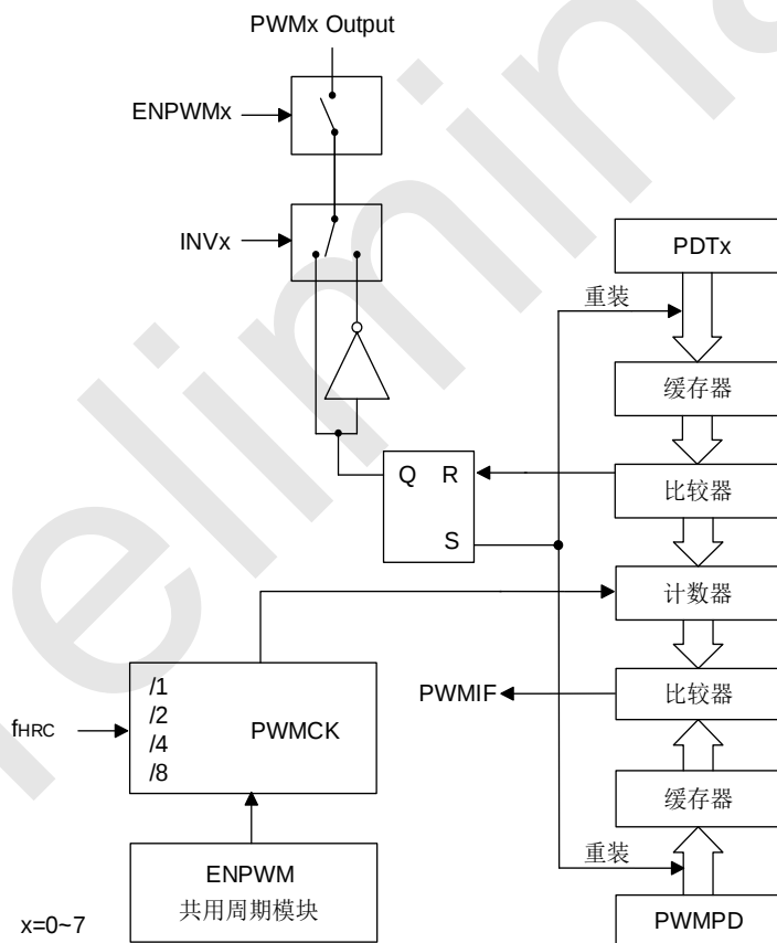
SC92F859X PWM 结构框图
