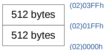
SC92F859X EEPROM Sector 分区示意
