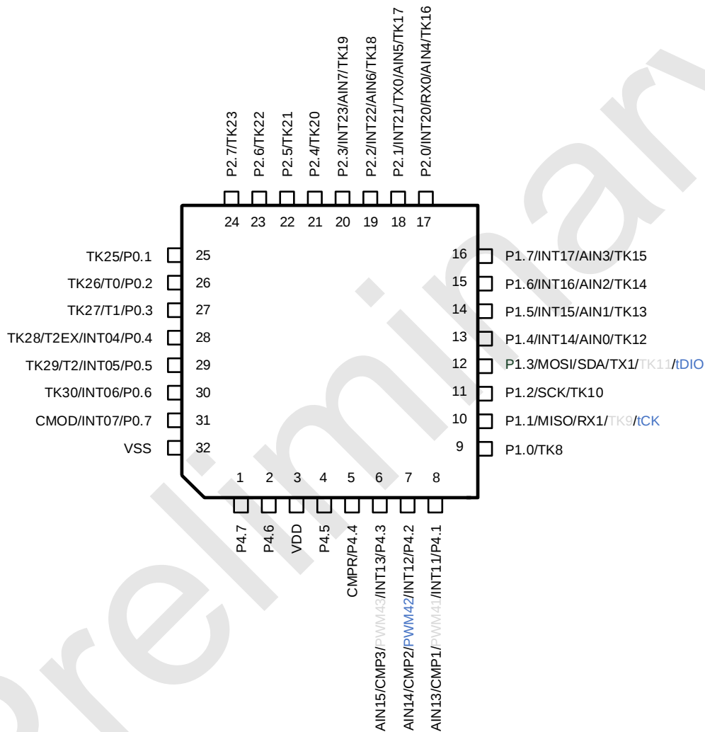
32PIN 管脚配置图
