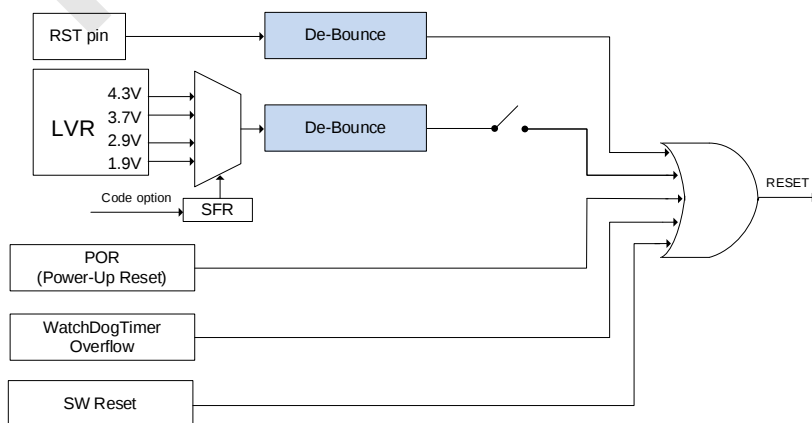
SC92F859X 复位电路图
