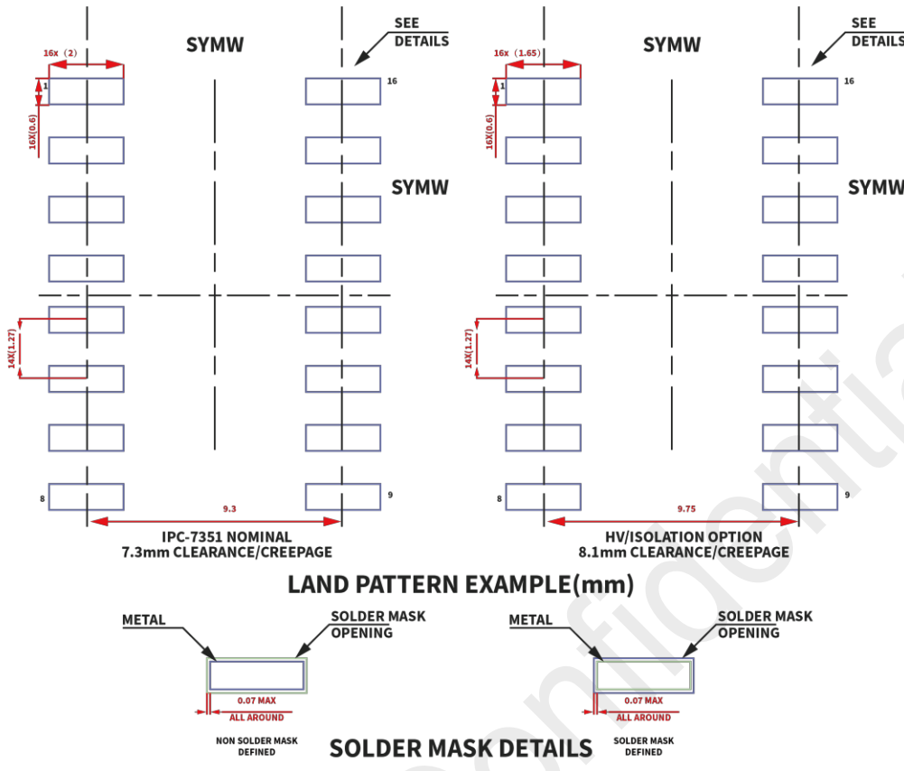
图 19. SOIC-16 封装板布局示例
