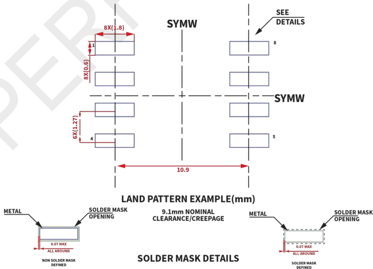
图 16. CMT10XXX SOW8L 封装
