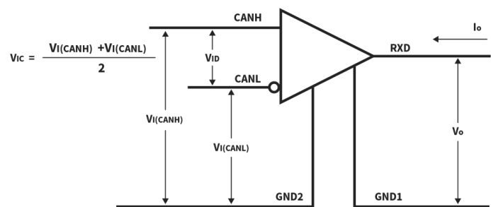
图 8. 驱动测试电路以及电压波形
