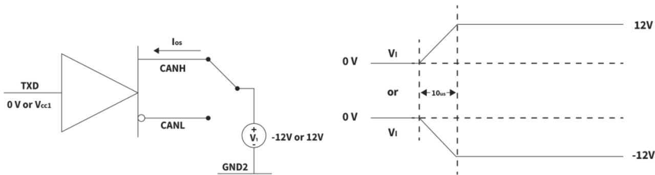
图 13. 驱动器短路电流测试电路及波形
