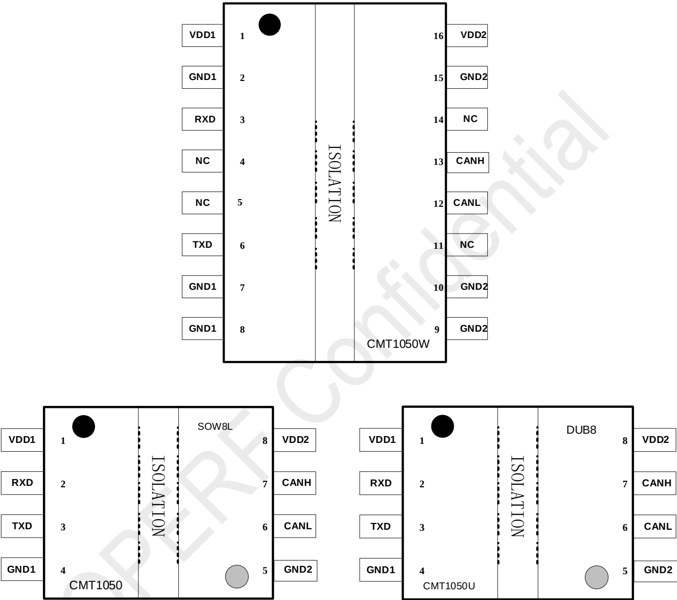
图 1. CMT1050X 引脚图
