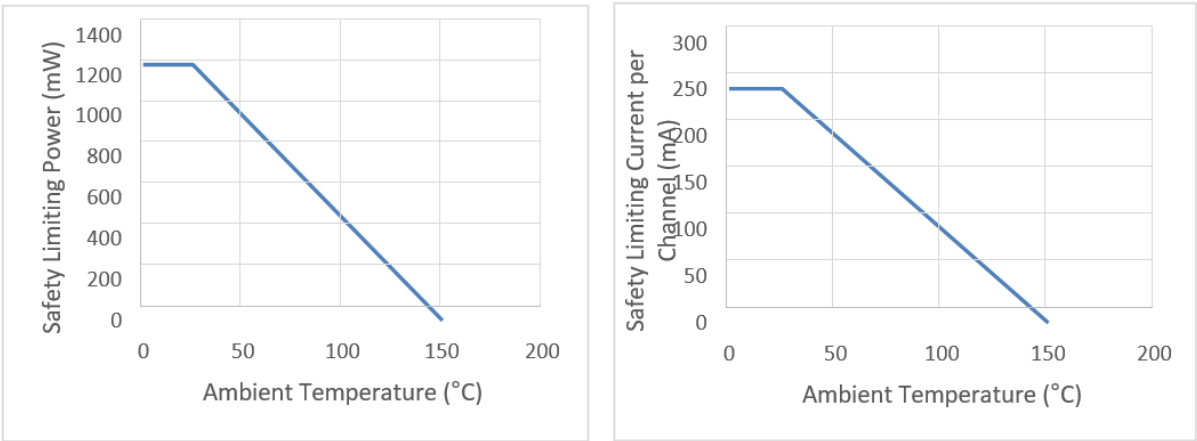
图 15. CMT10XXX 热降额曲线
