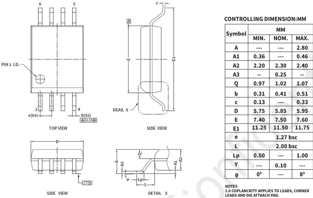
图 16. CMT10XXX SOW8L 封装
