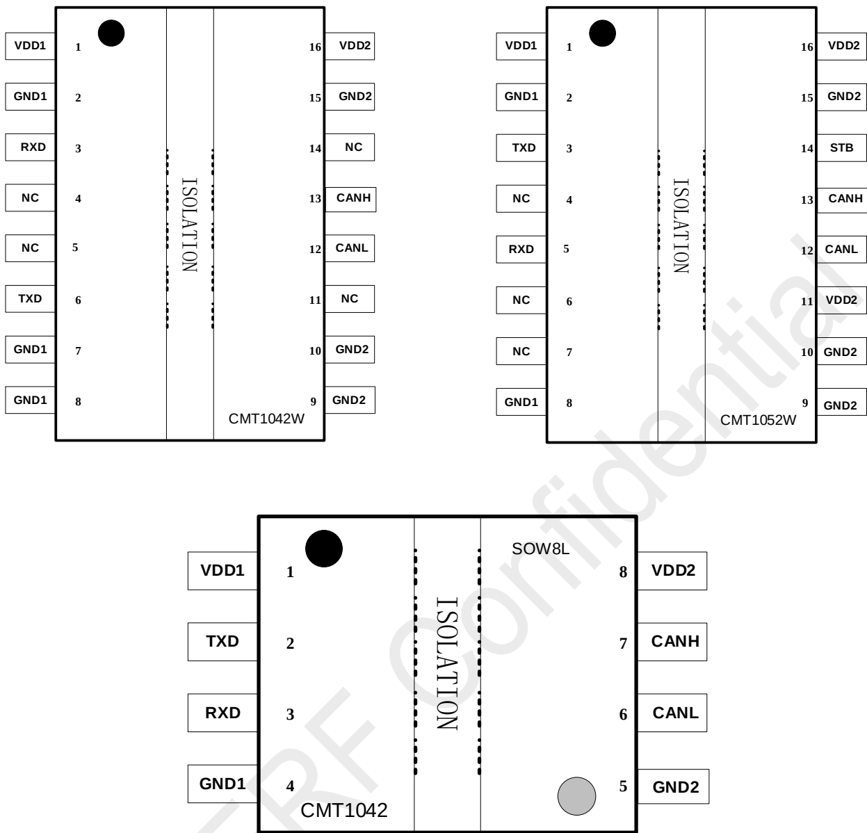
图 2. CMT1042W / CMT1052W 引脚图
