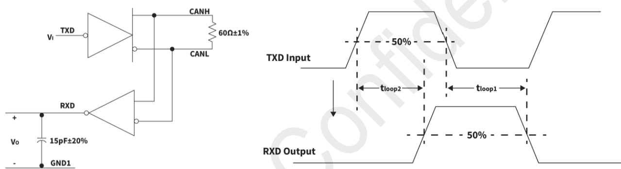
图 11. t_{\text{Loop}} 测试电路和电压波形
