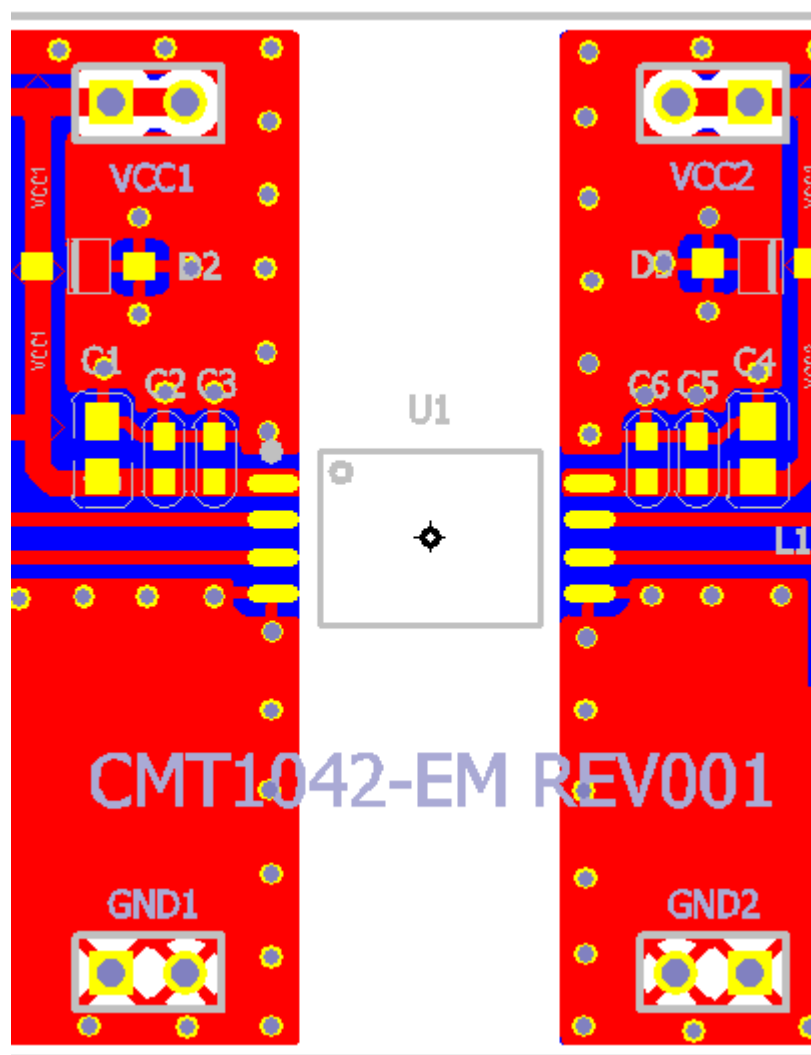
图 4.推荐布局指南（顶层）
