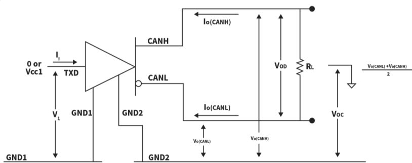
图 5. 驱动电压，电流指标定义
