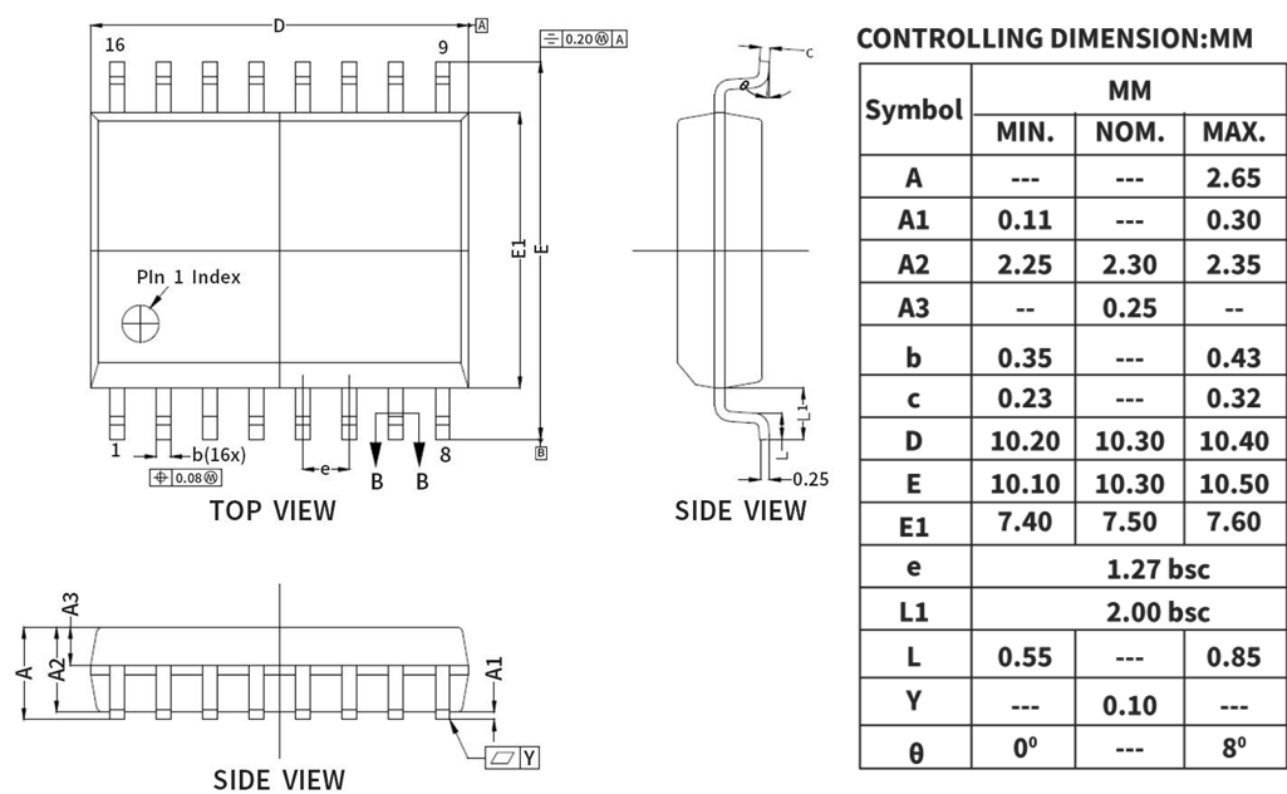
图 18. CMT10XXX SOIC 16 封装外形和尺寸
