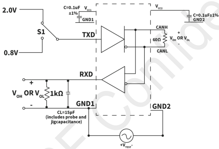
图 14. 共模瞬态抑制(CMTI)测量电路
