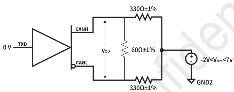
图 7. 驱动器 V_{OD} 电压测试电路（带共模负载）
