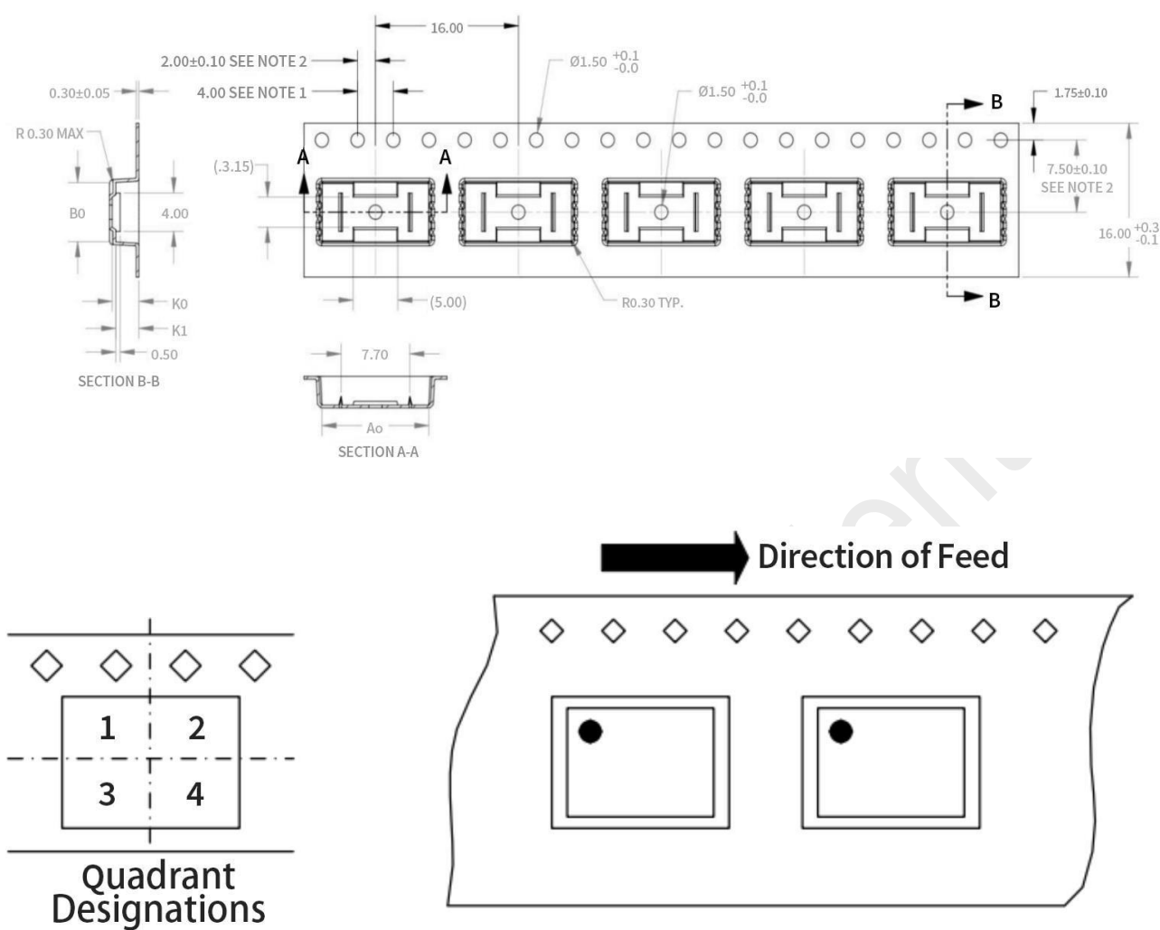
Figure 21. CMT10XXX SOIC-8 卷带信息
