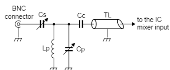
a. Schematic 1
