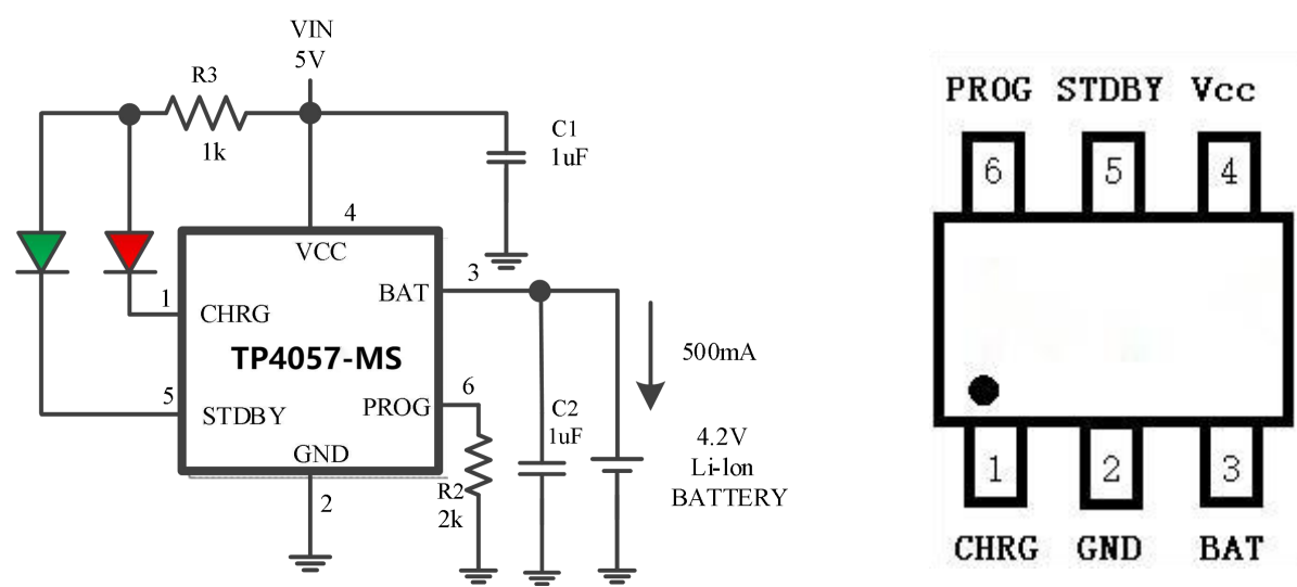
600mA 单节锂离子电池充电器
