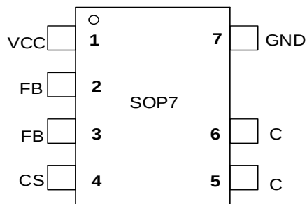
图 2 管脚封装图
