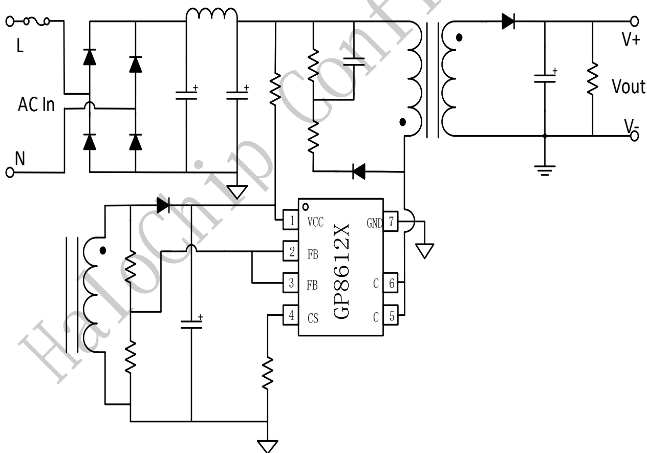
图 1 GP8612X 典型应用图
