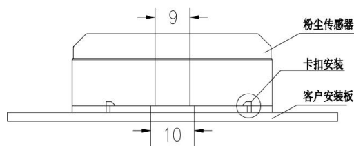
卡扣安装
