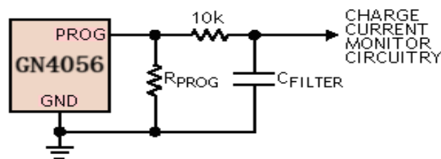
图2：隔离PROG 引脚上的容性负载和滤波电路
