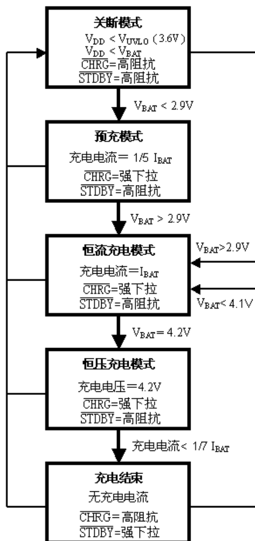
图1：一个典型充电循环的状态图
