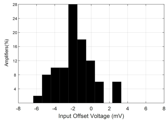
Fig.8-6. Offset Voltage
